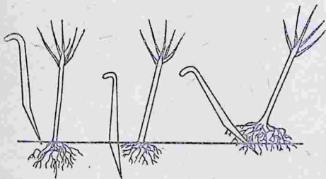
Р и с. 21. Схема работы шацким ломом.
