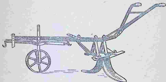
Рис. 22. Конный плуг для выкопки саженцев конструкции Оболянского питомника.
