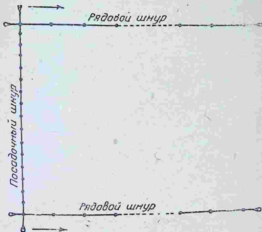
Рис. 17. Схема разбивки участка шнурами при посадке подвоев. Метки на рядовых шнурах отмечают пункты накладки посадочных шнуров, метки на посадочных шнурах — места посадки подвоев.
