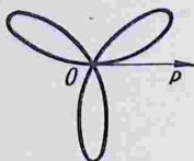
Р и с. 3. Трехлепестковая роза
