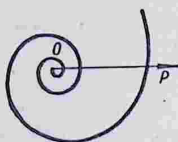
Р и с. 1. Логарифмическая спираль
