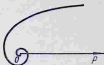
Р и с. 2. Гиперболическая спираль
