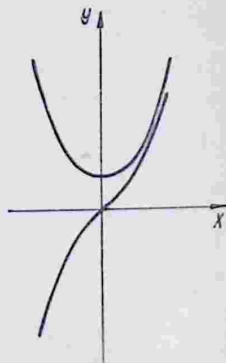
Р и с. 4. Графики гиперболических функций:
