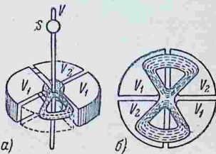
Рис. 79. Квадрантный электрометр.
