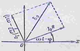
Рис. 309. Векторная диаграмма для цепи переменного тока с самоиндукцией и емкостью.
