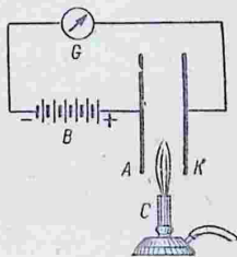
Рис. 150. Проводимость воздуха вблизи пламени.
