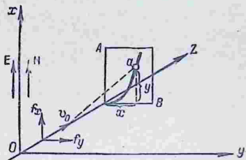
Рис. 275. Схема метода парабол.
