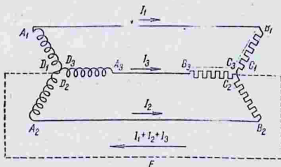
Рис. 326. Схема соединения звездой.
