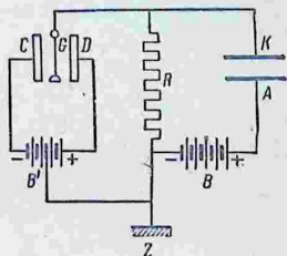
Рис. 153. Измерение малых токов методом постоянного отклонения.
