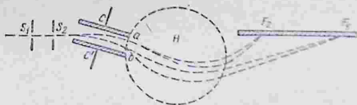
Рис. 276. Масс-спектрограф.
