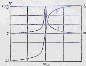
Рис. 308. Зависимость силы тока (1) и сдвига фаз (2) от частоты.
