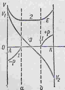
Рис. 156. Распределение между электродами: 1 — объемных зарядов \rho ; 2 — напряженности поля E ; 3 — потенциала.
