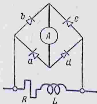
Рис. 324. Включение выпрямителей для измерения силы переменного тока.
