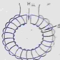
Рис. 218. Напряженность магнитного поля H_{\text{щ}} в щели равна магнитной индукции B в ферромагнетике.
