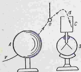
Рис. 44. Опыт с цилиндром Фарадея.
