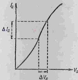
Рис. 357. Характеристика трехэлектродной лампы.
