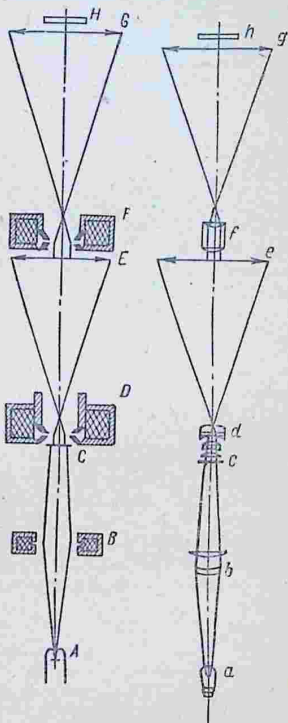
Рис. 286. Схемы микроскопов: электронного (слева) и оптического.
