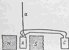
Рис. 302. Схема флюксметра.
