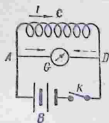
Рис. 296. Обнаружение экстратока размыкания.
