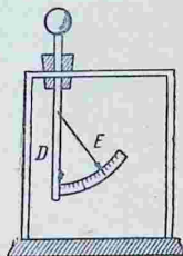
Рис. 4. Электрометр.
