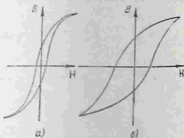
Рис. 223. Петля гистерезиса для: а — „мягкого“ материала; б — „жесткого“ материала.
