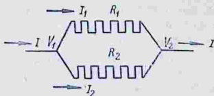
Рис. 88. Параллельное соединение проводников.
