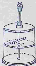
Рис. 7. Крутильные весы Кулона.
