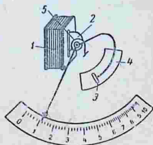
Рис. 255. Технический амперметр постоянного тока.
