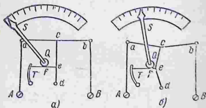
Рис. 89. Схема теплового измерительного прибора.
