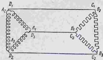
Рис. 327. Схема соединения треугольником.
