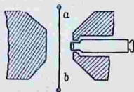
Рис. 258. Струнный гальванометр.
