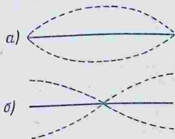
Рис. 346. Распределение амплитуды силы тока (а) и амплитуды электрической напряженности (б) вдоль диполя.
