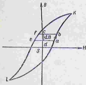
Рис. 300. К подсчету работы перемагничивания.
