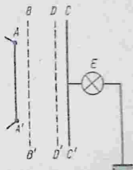
Рис. 167. Схема метода определения ионизационных потенциалов.
