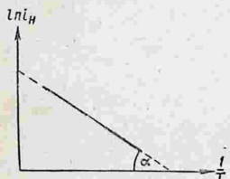
Рис. 140. Линейная зависимость логарифма тока насыщения от 1/T .
