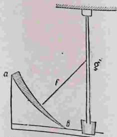
Рис. 3. Электрический указатель Г. В. Рихмана.
