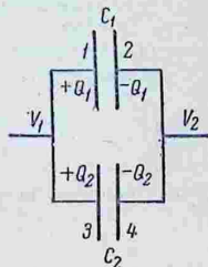
Рис. 69. Параллельное соединение конденсаторов.
