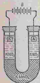
Рис. 146. Метод наблюдения подвижности ионов.
