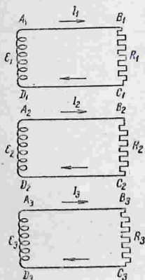
Рис. 325. Схема возбуждения трехфазного тока.
