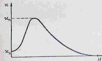
Рис. 221. Зависимость для ферромагнетика коэффициента намагничивания \kappa от напряженности поля H .
