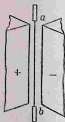
Рис. 78. Струнный электрометр.
