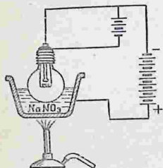
Рис. 149. Способ наблюдения электролитической проводимости стекла.
