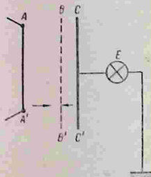
Рис. 166. Схема метода Франка и Герца определения ионизационных потенциалов.
