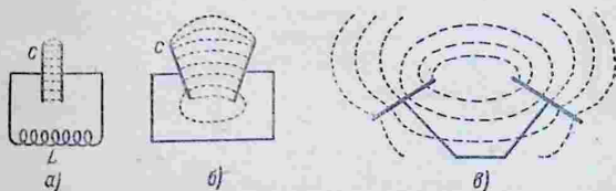
Рис. 343. Колебательные контуры различной степени открытости.
