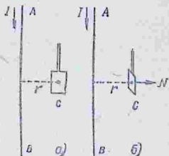
Рис. 186. Определение напряженности поля с помощью рамки.
