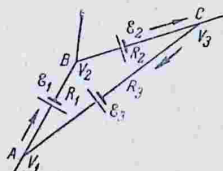
Рис. 112. Замкнутый контур ABCA .
