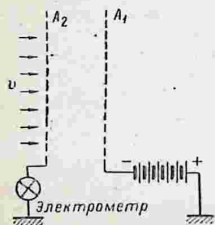
Рис. 157. Схема простейшего способа определения подвижности ионов.
