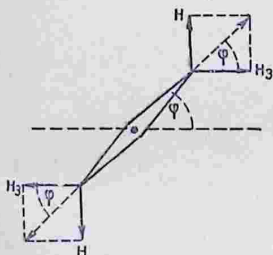
Рис. 252. К определению положения равновесия стрелки тангенс-гальванометра.
