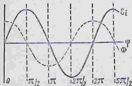
Рис. 294. Графики изменения потока индукции \Phi и электродвижущей силы индукции \mathcal{E}_i во вращающейся рамке.
