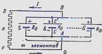
Рис. 117. Параллельное соединение элементов в батарею.
