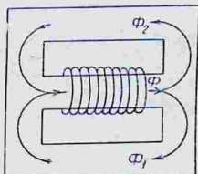
Рис. 246. Параллельное разветвление магнитной цепи.
