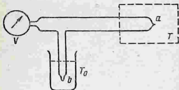
Рис. 130. Схема измерения температуры с помощью термопары.
