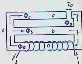
Рис. 249. Электромагнит с разветвленной магнитной цепью.
