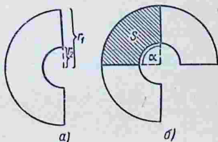
Рис. 74. Пластины конденсатора переменной емкости.
