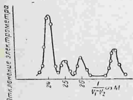
Рис. 279. Кривая для изотопов магния.
