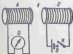
Рис. 289. Возбуждение в соленоиде индукционного тока при включении или выключении тока в соседнем соленоиде.
