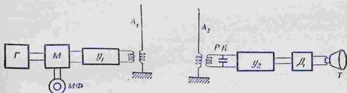
Рис. 359. Схема передающей и принимающей радиостанций.
