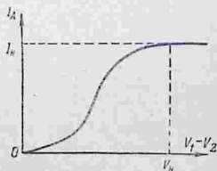
Рис. 138. Зависимость анодного тока I_A от разности потенциалов V_1 - V_2 между катодом и анодом.
