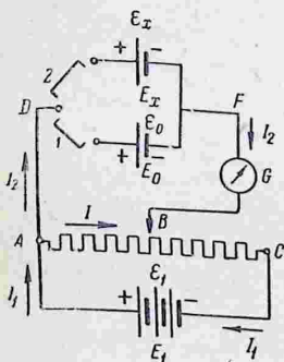
Рис. 118. Схема компенсационного метода определения электродвижущей силы элемента.
