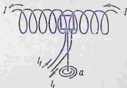
Рис. 207. Рамка с током внутри соленоида.
