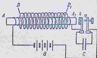
Рис. 317. Индукционная катушка.
