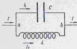
Рис. 334. Цепь из параллельно соединенных емкости C и самоиндукции L .
