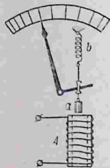
Рис. 254. Амперметр Доливо-Добровольского.
