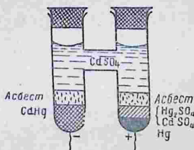
Рис. 119. Нормальный элемент.
