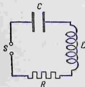
Рис. 307. Цепь с омическим сопротивлением R , самоиндукцией L и емкостью C .
