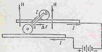
Рис. 193. Обнаружение силы \Delta f , действующей на проводник с током во внешнем магнитном поле H .
