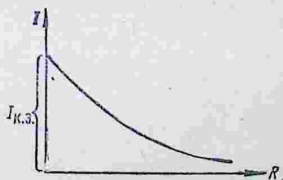
Рис. 108. Зависимость силы тока от внешнего сопротивления.
