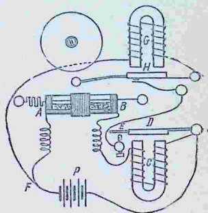
Рис. 354. Схема приемника А. С. Попова.
