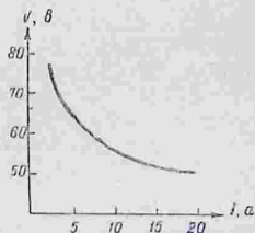
Рис. 173. Падающая вольт-амперная характеристика дугового разряда.
