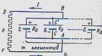
Рис. 117. Параллельное соединение элементов в батарею.
