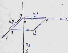
Рис. 341. К определению первой системы уравнений Максвелла.
