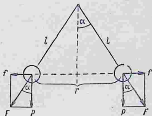
Рис. 10. Силы, действующие на наэлектризованные шары.
