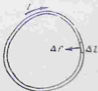
Рис. 201. Сила, действующая на элемент \Delta l контура с током, расположенного перпендикулярно напряженности магнитного поля.
