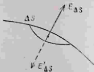
Рис. 47. Напряженность поля, образуемого элементом поверхности заряженного проводника.
