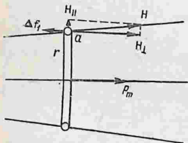
Рис. 204. Контур с током в неоднородном магнитном поле.
