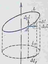
Рис. 209. К расчету циркуляции вектора магнитной напряженности H .
