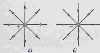
Рис. 16. Линии напряженности точечного заряда: а — положительного; б — отрицательного.
