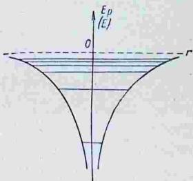
Рис. 100. Энергетические уровни электрона в кулоновом поле.
