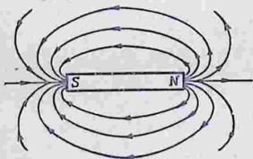
Рис. 228. Линии напряженности постоянного прямого магнита.
