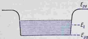
Рис. 101. Уровни энергии электронов в кристалле.
