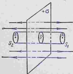
Рис. 27. К подсчету напряженности поля бесконечной плоскости.
