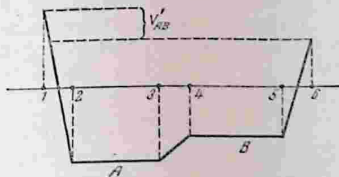
Рис. 124. Потенциальная яма двух соприкасающихся металлов.
