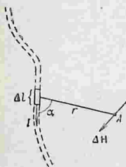
Рис. 187. Элемент тока \Delta l создает в точке A напряженность магнитного поля \Delta H , перпендикулярную к плоскости, содержащей \Delta l и радиус-вектор r .
