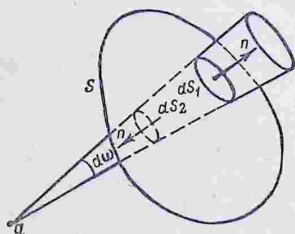
Рис. 25. К определению потока от заряда, находящегося вне замкнутой поверхности.
