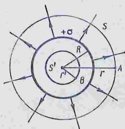
Рис. 29. К определению напряженности поля заряженной сферы.
