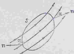
Рис. 185. Поток линий напряженности через замкнутую поверхность.
