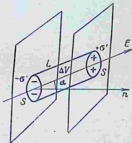
Рис. 55. К определению значения вектора поляризации P .
