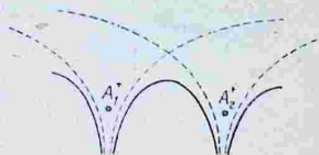
Рис. 98. Потенциальные кривые вблизи положительных зарядов.
