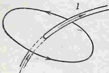
Рис. 208. Направление обхода тока при положительной циркуляции.
