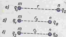
Рис. 8. К обоснованию закона Кулона.
