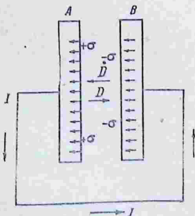
Рис. 338. Возникновение тока смещения между обкладками конденсатора.
