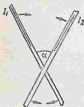
Рис. 200. Взаимодействие двух прямых токов, текущих под углом \alpha друг к другу.
