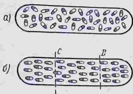
Рис. 6. Поляризация диэлектрика.
