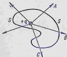
Рис. 23. Пересечение линиями напряженности произвольной замкнутой поверхности.
