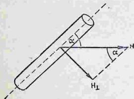
Рис. 229. Составляющая напряженности поля H , перпендикулярная оси магнита.
