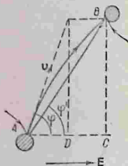
Рис. 169. К определению пути электрона между двумя столкновениями.
