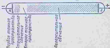
Рис. 171. Тлеющий разряд.
