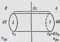
Рис. 126. К подсчету давления электронного газа.
