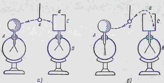
Рис. 43. Опыт с цилиндром Фарадея.
