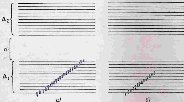
Рис. 136. Зоны дозванных состояний электронов в кристалле: а) диэлектрика; б) металла.
