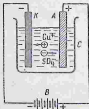
Рис. 142. Движение ионов \text{Cu}^{++} и \text{SO}_4^{--} при электролитической проводимости раствора медного купороса.
