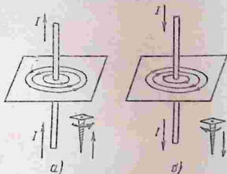
Рис. 179. Направление линий напряженности магнитного поля прямого тока.
