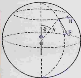
Рис. 350. Направление векторов E и H в волновой зоне диполя.
