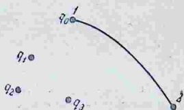
Рис. 34. Перемещение заряда q_0 в поле системы зарядов q_1, q_2, \dots, q_n .
