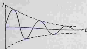
Рис. 330. Затухающие колебания.
