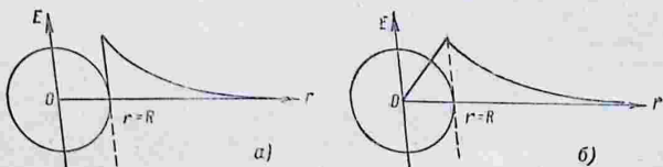
Рис. 30. Напряженность поля: а — поверхностно заряженной сферы; б — объемно заряженной сферы.
