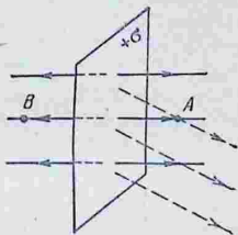
Рис. 26. Линии напряженности поля бесконечной плоскости.
