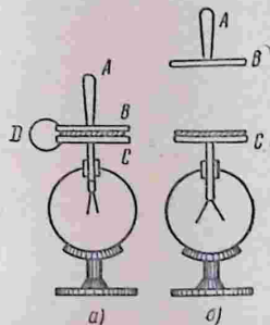
Рис. 121. Обнаружение контактной разности потенциалов.
