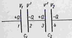
Рис. 68. Последовательное соединение конденсаторов.
