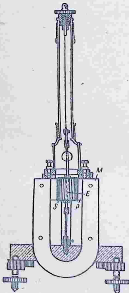
Рис. 257. Зеркальный гальванометр.
