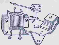
Рис. 323. Схема индукционного амперметра.
