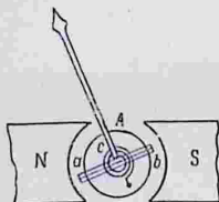
Рис. 256. Схема гальванометра с подвижной рамкой.
