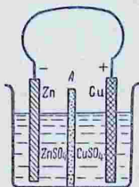
Рис. 104. Элемент Даниэля.
