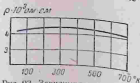
Рис. 93. Зависимость удельного сопротивления \rho манганина от абсолютной температуры T .
