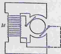
Рис. 314. Схема динамомашины с последовательным возбуждением.
