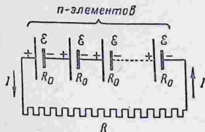
Рис. 116. Последовательное соединение элементов в батарею.
