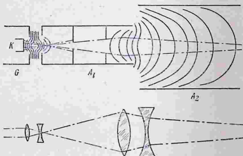
Рис. 284. Фокусирующая система осциллографа.
