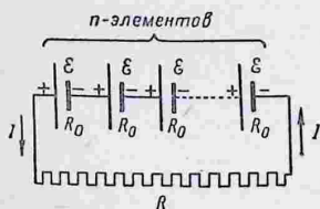
Рис. 116. Последовательное соединение элементов в батарее.
