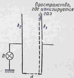
Рис. 158. Схема метода определения подвижности ионов.
