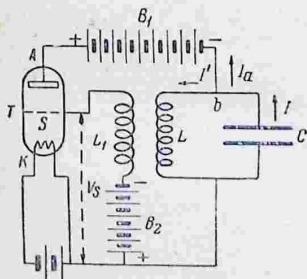
Рис. 337. Схема возбуждения незатухающих колебаний с помощью трехэлектродной лампы.
