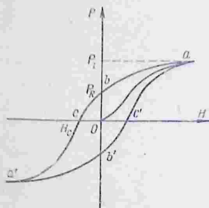
Рис. 222. Петля гистерезиса.
