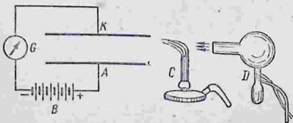
Рис. 151. Увлечение ионов потоком воздуха.
