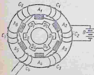
Рис. 311. Схема генератора переменного тока с неподвижными обмотками.
