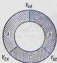
Рис. 125. Замкнутая цепь из трех металлов.
