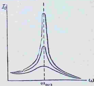
Рис. 333. Резонансные кривые силы тока I .
