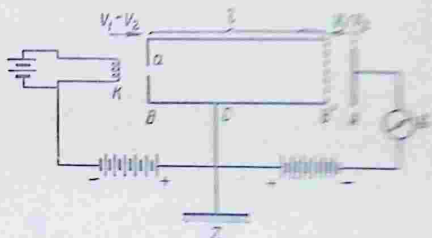
Рис. 161. Схема метода определения средней длины свободного пути электронов.
