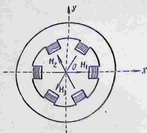
Рис. 328. Кольцевая магнитная цепь.
