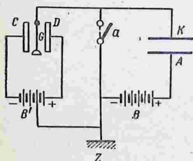
Рис. 152. Измерение малых токов методом натекания.
