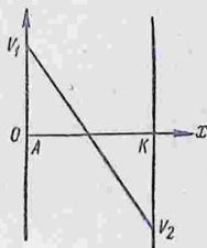
Рис. 155. Распределение потенциала V между электродами при отсутствии ионизации.
