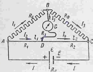
Рис. 115. Схема мостика Уитстона.
