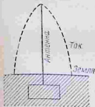
Рис. 355. Свободные колебания простейшей вертикальной антенны.
