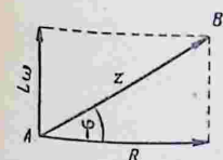
Рис. 306. Графическое определение полного сопротивления z в цепи переменного тока с самоиндукцией по омическому сопротивлению R и индуктивному сопротивлению L\omega .
