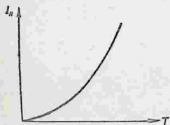
Рис. 139. Зависимость тока насыщения I_n от температуры T катода.
