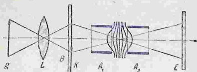
Рис. 285. Электронно-оптический преобразователь.
