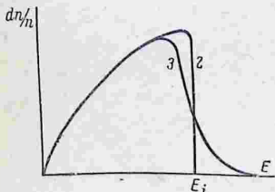
Рис. 103. Распределение электронов по энергиям: 2 — при T=0 ; 3 — при T \neq 0 .
