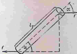
Рис. 230. К определению момента сил, действующего на магнит.
