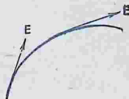
Рис. 15. Линия напряженности.
