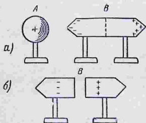
Рис. 5. Электризация наведением.
