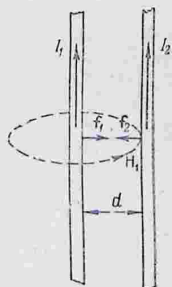
Рис. 199. Взаимодействие двух прямолинейных бесконечных токов.
