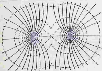
Рис. 38. Поверхности уровня потенциала (пунктирные линии) и линии напряженности (сплошные линии) двух точечных одноименных зарядов.
