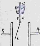
Рис. 77. Электро-скоп с заряженными пластинками.
