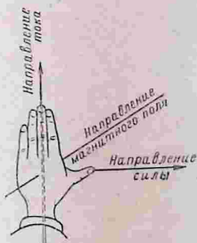
Рис. 197. Правило левой руки.
