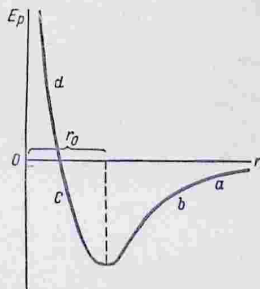
Рис. 144. Зависимость потенциальной энергии E_p от расстояния r .
