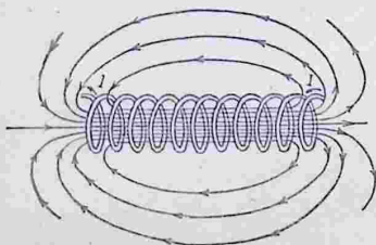
Рис. 181. Направление линий напряженности магнитного поля соленоида.
