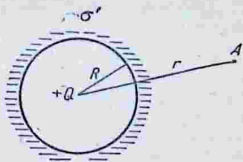
Рис. 56. Влияние диэлектрика на поле заряженного шара.
