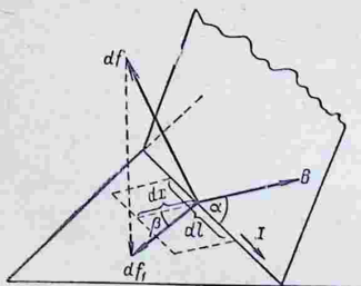
Рис. 241. К подсчету работы перемещения участка с током dl в магнитном поле.
