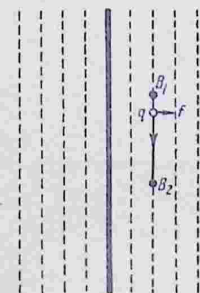
Рис. 37. Поверхности уровня потенциала бесконечной заряженной плоскости.
