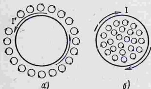
Рис. 239. Сложение молекулярных токов на поверхности полости.
