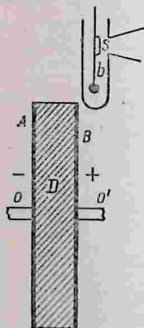
Рис. 265. Схема опыта Эйхенвальда по определению магнитного поля движущегося диэлектрика.
