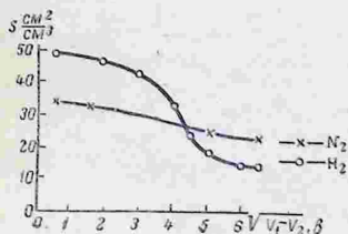
Рис. 162. Зависимость от скорости электронов эффективного сечения S молекул \text{H}_2 и \text{N}_2 , находящихся в 1 \text{ см}^3 при 0^\circ \text{C} и при давлении 1 мм. Нг.
