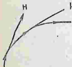
Рис. 178. Линии магнитной напряженности.
