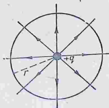
Рис. 21. К выводу теоремы Остроградского — Гаусса.
