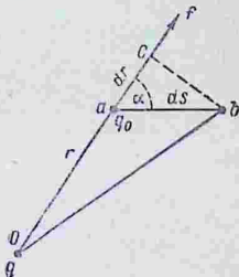
Рис. 32. К определению работы перемещения заряда q_0 на пути ds .
