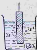
Рис. 127. Переход ионов цинка в раствор серной кислоты.
