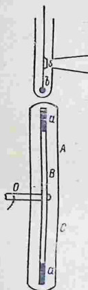
Рис. 264. Схема опыта Эйхенвальда.
