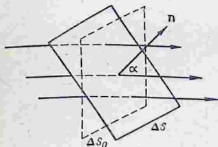
Рис. 60. Площадка \Delta S , расположенная наклонно к линиям электростатической индукции \mathbf{D} .
