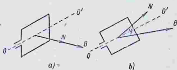
Рис. 293. Рамка, вращающаяся во внешнем магнитном поле.
