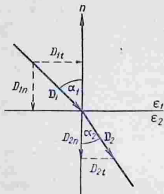
Рис. 62. Преломление линий индукции на границе двух диэлектриков.
