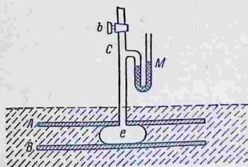
Рис. 58. К расчету дополнительного давления.
