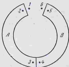
Рис. 122. К объяснению контактной разности потенциалов.
