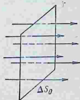
Рис. 19. Площадка \Delta S_0 , перпендикулярная к линиям напряженности.
