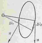
Рис. 211. К расчету циркуляции H по замкнутому контуру, не охватывающему ток.
