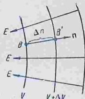
Рис. 40. Нормаль n к двум близким уровням потенциала.
