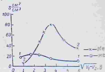
Рис. 163. Зависимость от скорости электронов эффективного сечения S атомов He и Ne, находящихся в 1 см³ при 0°C и при давлении 1 мм Hg.
