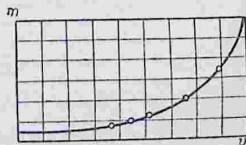
Рис. 272. Зависимость массы электрона от скорости.
