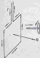
Рис. 177. Направление положительной нормали к рамке с током.
