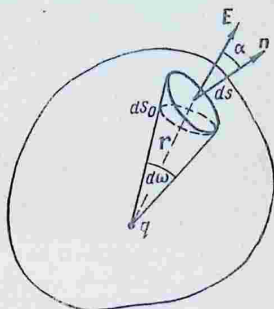
Рис. 24. К более точному выводу теоремы Остроградского — Гаусса.
