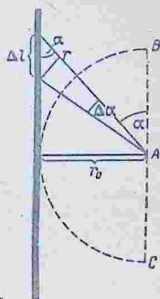
Рис. 188. К подсчету напряженности магнитного поля прямого тока.
