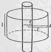
Рис. 31. К определению напряженности поля заряженного цилиндра.
