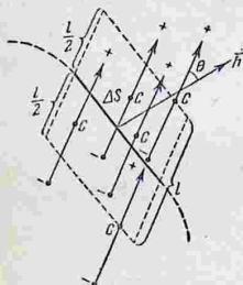
Рис. 64. К подсчету связанного заряда.
