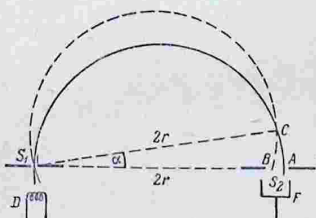
Рис. 278. Схема отклонения частиц в поперечном магнитном поле.
