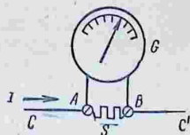
Рис. 90. Включение шунта S .
