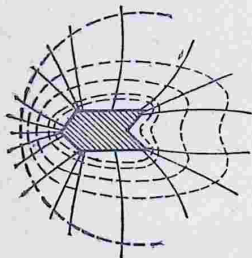
Рис. 46. Расположение эквипотенциальных поверхностей (пунктирные линии) и линий напряженности (сплошные линии) у тела с выступом и впадиной.
