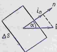
Рис. 83. К определению нормальной составляющей плотности тока i_n .
