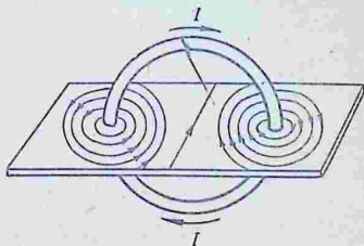
Рис. 180. Направление линий напряженности магнитного поля кругового тока.
