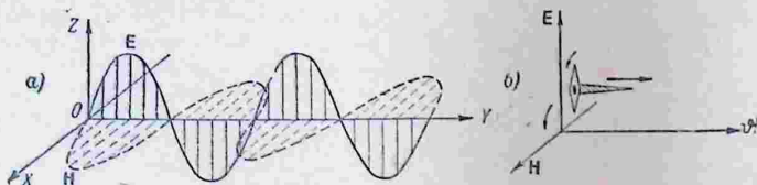
Рис. 352. Электромагнитная волна.
