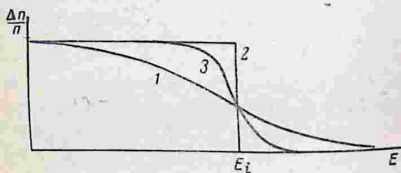
Рис. 102. Распределение электронов по энергетическим уровням: 1 — по Большцману при T \neq 0 ; 2 — по Ферми при T = 0 ; 3 — по Ферми при T \neq 0 .
