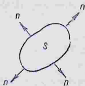
Рис. 85. Внешние нормали к замкнутой поверхности S .
