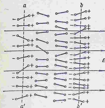
Рис. 54. Появление объемных зарядов при поляризации неоднородного диэлектрика.
