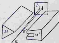
Рис. 215. Схема опыта Штерна и Герлаха.
