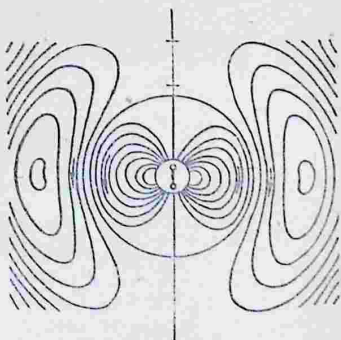
Рис. 348. Линии напряженности около диполя.
