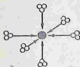
Рис. 143. Молекулы воды, окружающие ион.
