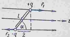
Рис. 49. Диполь во внешнем неоднородном поле.
