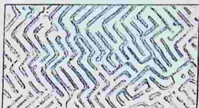
Рис. 224. Области намагничивания.
