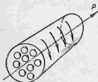
Рис. 217. Сложение молекулярных токов в намагниченной среде.
