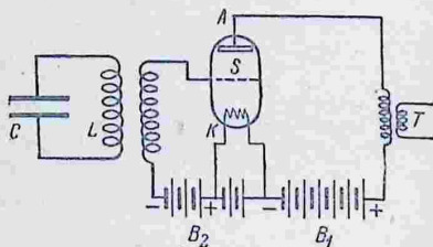
Рис. 356. Схема усиления электромагнитных колебаний.
