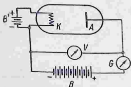
Рис. 137. Наблюдение термоэлектронной эмиссии с помощью катодной лампы.
