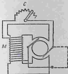
Рис. 315. Схема динамомашины с параллельным возбуждением.
