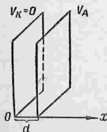
Рис. 160. К выводу формулы Богуславского — Ленгмюра.
