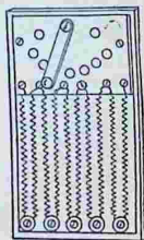
Рис. 94. Реостат со скользящим контактом.
