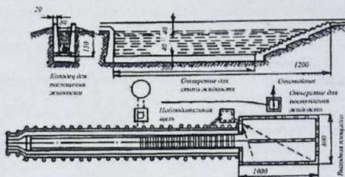
Рис. 170. План ванны для купания овец
