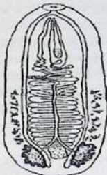
Рис. 13. Catotropis verrucosa
