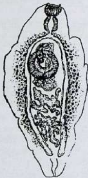
Рис. 2. Parafasciolopsis fasciolaemorpha
