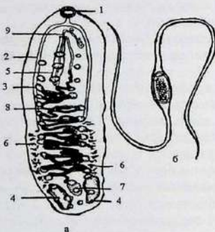
Рис. 12. Notocotylus attenuatus :
