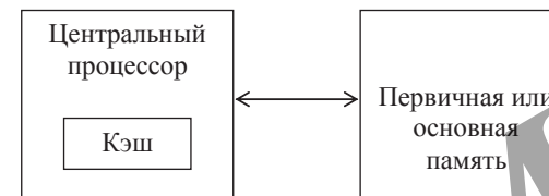
Рис. 3.24. Внутренний кэш (кэш 1 уровня) 20
