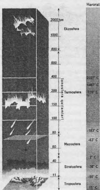
22-rasm. Atmosfera tuzilishi
