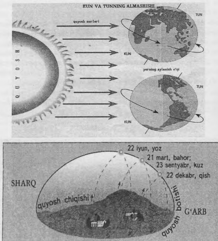
17-rasm. Yerning quyoshga nisbatan holati
