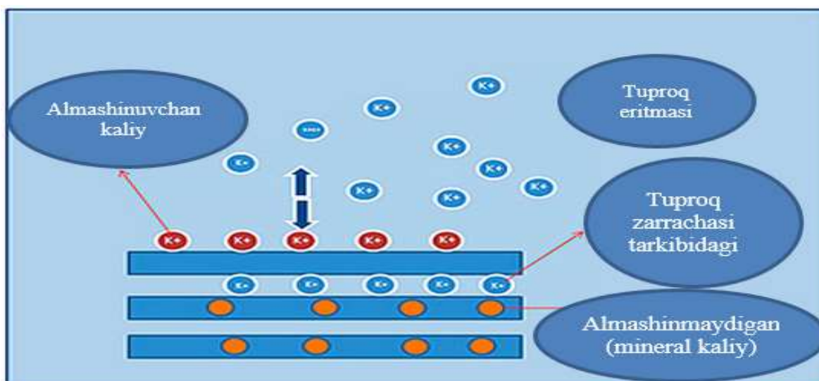
23-rasm. Tuproqdagi kaliy fraksiyalari.
