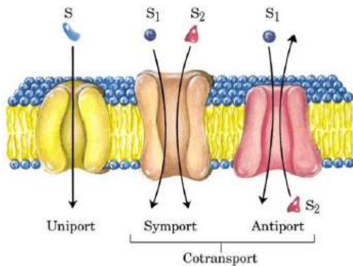
8 - rasm. Simport va antiport mexanizimi.
