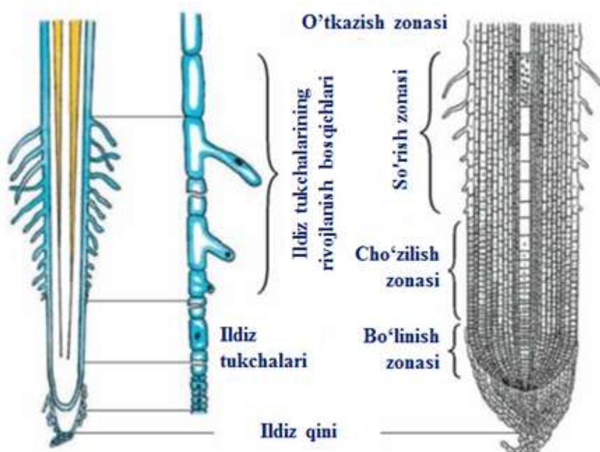
5-rasm. Ildiz tuzilishi.
