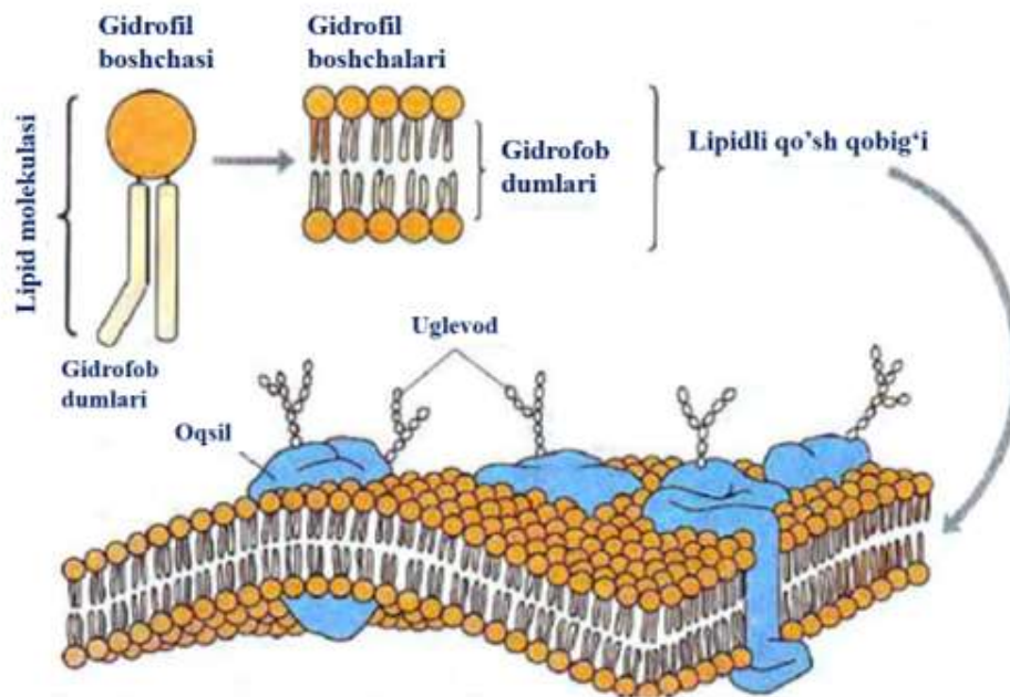
6-rasm. Suyuq-mozaika membrana modeli.
