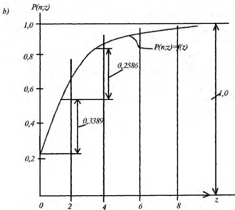
12.2-rasm. Ehtimollik (a) va kumulativ (b) ehtimollikning mustahkamlik grafiklari.
