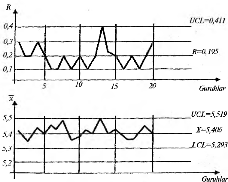
12.1-rasm. Plastinaning qalinligi uchun ( \bar{X} - R ) nazorat kartasi.
