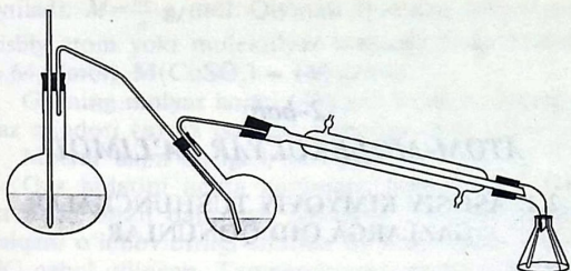
19-rasm. Suv bug'i bilan haydash asbobi.
