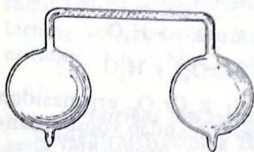
26-rasm. \text{NO}_2 bilan \text{N}_2\text{O}_4 o'rtasidagi muvozanatga temperaturaning ta'siri.
