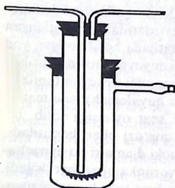
16-rasm. Vakuumda sublimatsiya qilish asbobi.
