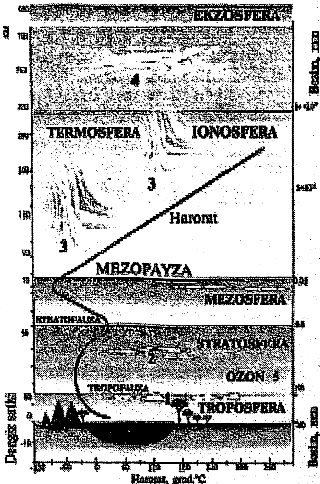
Atmosferaning vertikal tuzilishi namosi 1-ko'ndalang va poytaxt bulutlari; 2-stratosferada bulutlar; 3-quyi ko'ndalangdagi qalb yuq'dalok; 4-yuqori ko'ndalangdagi qalb yuq'dalok; 5-ozon mintaqasi eng ko'p qatlam.
