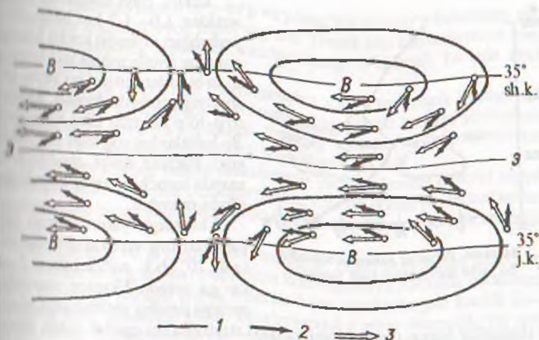
13-rasm. Passatlar zonasidagi havo oqimlari sxemasi.
