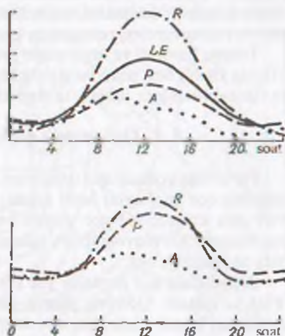
23 - r a s m. Issiqlik balansini tashkil etuvchilarining sutkalik o'zgarishi. a) Sankt-Peterburg; b) O'rta Osiyo chalacho'llari. Iyul.
