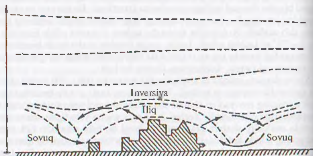
28-rasm. Kuchsiz shamol sharoitida rivojlanadigan shahar sirkulyatsiyasi.
