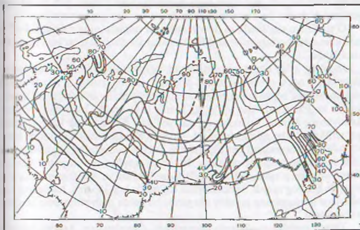
24-rasm. MDH hududidagi qor qoplaminin balandligi (sm).
