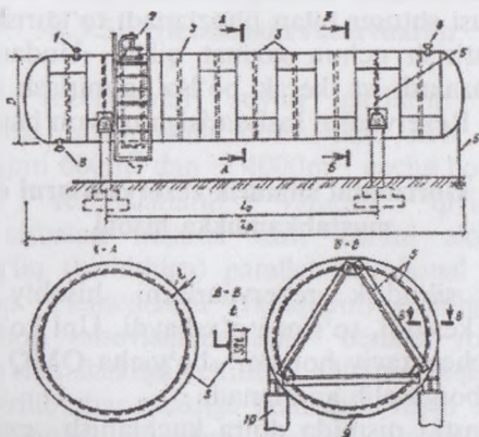
18.6-rasm. Gorizontal silindrik rezervuar: 1,4,8 – shtuser; 2 – koʻrish teshigi; 3 – bikirlik doirasi; 5 – tayanch diafragmasi.
