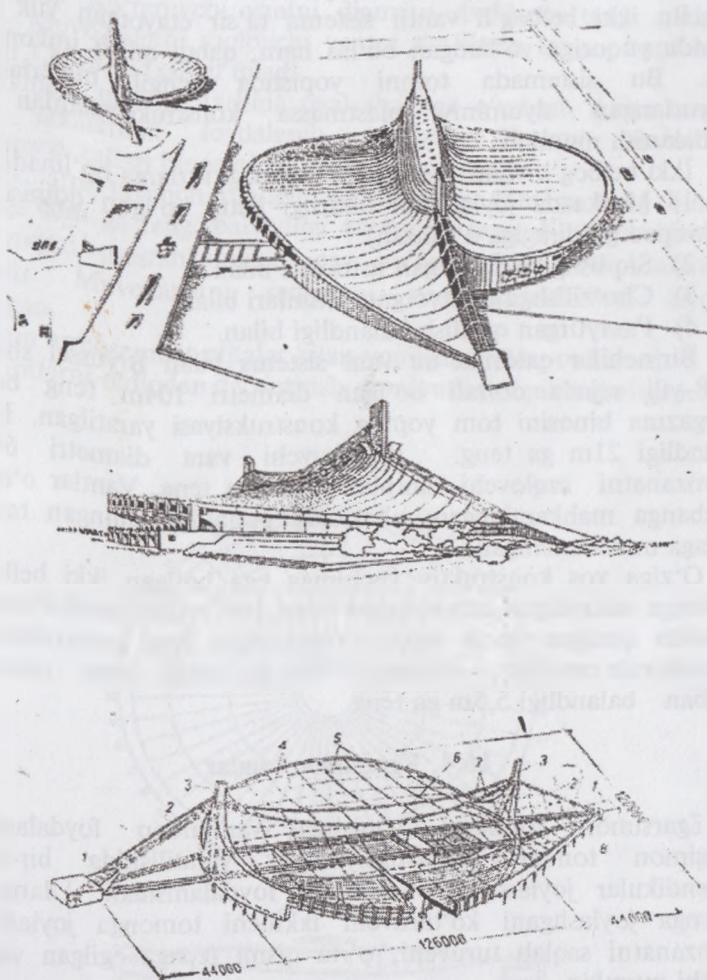
16.3-rasm. Tokio shahrida qurilgan sport kompleksi hinosi tom yopma konstruksiyasi.
