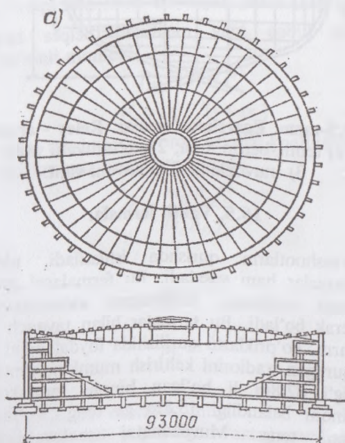
16.4-rasm. Ikki belbog'li vantli sistema Sankt - Peterburgdagi «Yubiley» sport saroyning tom yopma konstruksiyasi.
