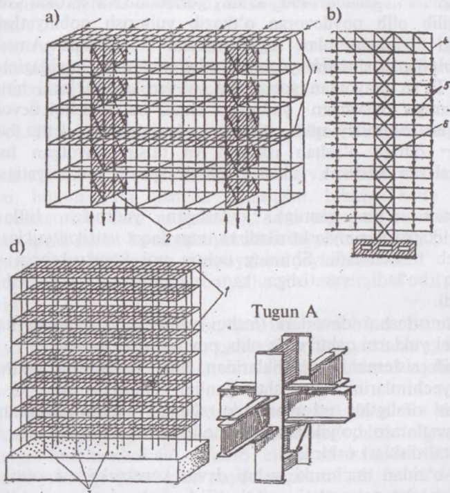
17.7-rasm. Baland binolarni sinchini sxemasi: a) bog'lovchi elementlar bilan; b) ramali; d) o'rta qismida yadrosi bilan. 1) gorizontall disklar; 2) vertikal disklar; 3) ramalar; 4) to'sin; 5) tortqich; 6) yadro.
