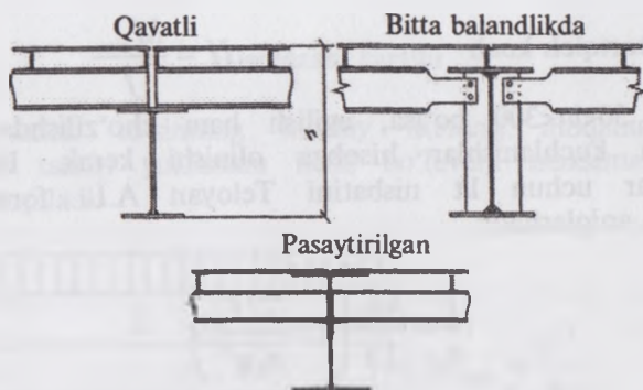
6.2-rasm. Murakkab to'sinli katakda to'sinlarni bir-biriga biriktirishi.
