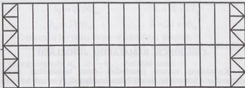
9.2-rasm. Fermani tepa tokchasi bo'yicha bog'lovchi elementlar tizimi.
