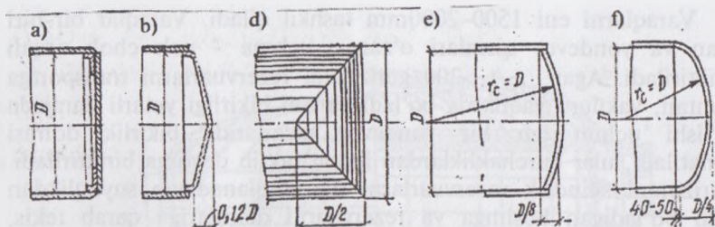
18.7-rasm. Gorizontaal silindrik rezervuarlar tublari.
