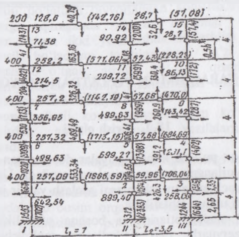
17.13-rasm. Ramalarni gorizontaal yukka hisobiy sxemasi.
