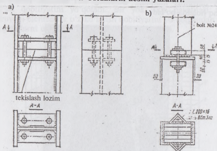
17.9-rasm. Ustunlarni kesim yuzalari.
