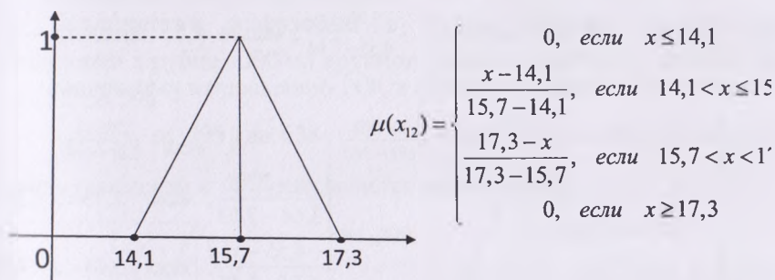
Рис. 3.11 - График функции принадлежности "Медь"
