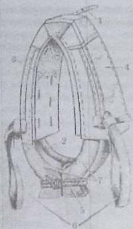
Рисунок 10. Хомут неразборный стандартный сельскохозяйственный: 1 — клещи; 2 — хомутина; 3 — хомутная подкладка; 4 — покрышка; 5 — супонье; 6 — пара гужей; 7 — горт
