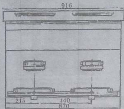
Рисунок 26. Общий вид двадцатирамочного улья
