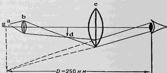
9-rasm. Mikroskopning optik sxemasi:
