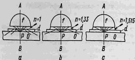
10-rasm. Optik mikroskopning obyektivi:
