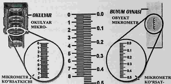
11-rasm. Obyekt-mikrometr va okulyar-mikrometr shkalasini taqqoslash. 2
