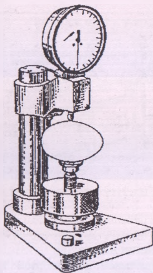
Рис. 7 Прибор для измерения упругой деформации яиц ПУД-1
