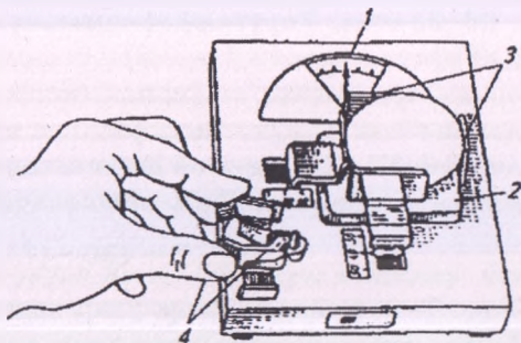
Рис. 6 Индексомер ИМ-1 для определения формы яиц: 1 — шкала индексомера; 2 — платформа прибора; 3 — упоры; 4 — рукоятки.
