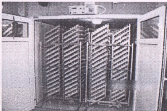
Рис. 17 Инкубатор ИП-36
