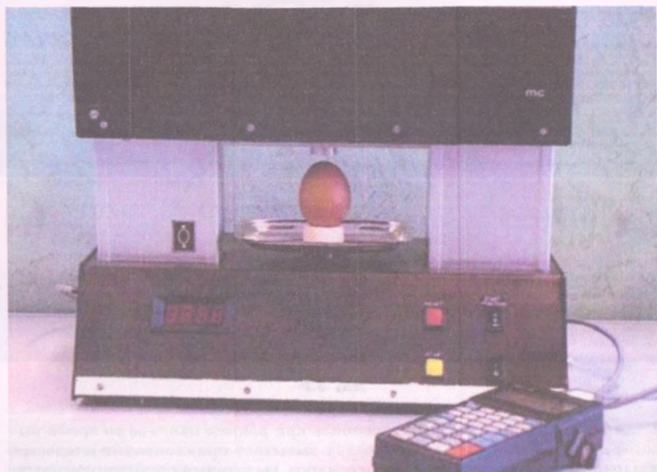
Ил. 35 Прибор для определения прочности скорлупы яиц BMP 2.1, подсоединенный к персональному компьютеру терминалу РТС-710
