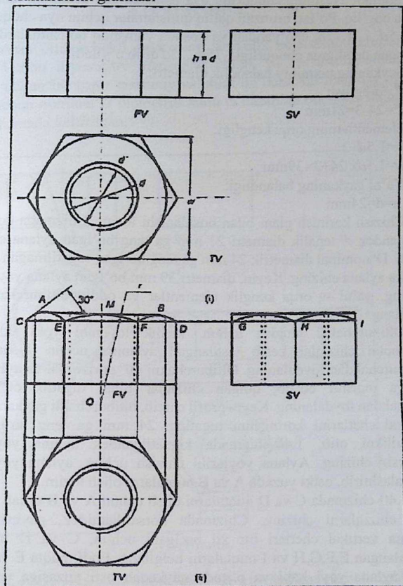
1.40-chizma. Oltiburchak gaykaning uchta ko'rinishi
