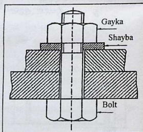
1. 29-a chizma. Bolt, gayka va shayba.
