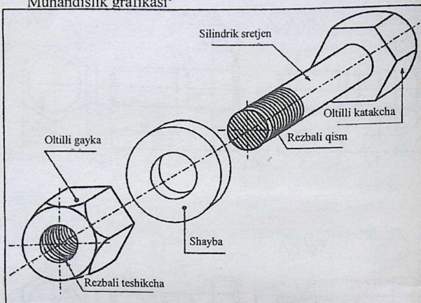
1. 29-a chizma. Bolt, gayka va shayba.
