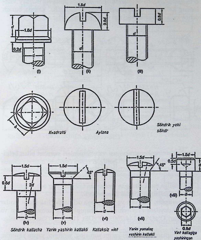
1.35-chizma. Turli kallakli vintlar.
