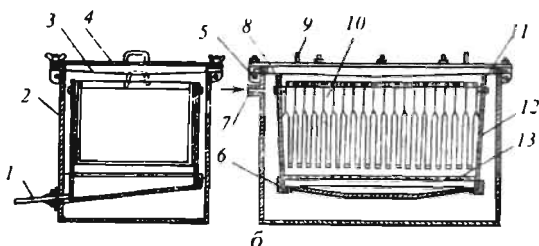
66-расм. Катта ҳажмдаги мумкатак рамкаларни жойлаштириб мум олишга мўлжалланган бугли мум эриткич: а – бугли мум эриткичининг умумий кўриниши; б – мум эриткичининг тузилиши:
