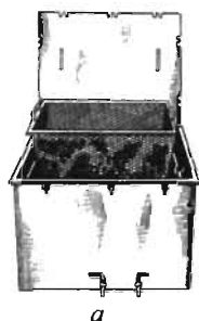
66-расм. Катта ҳажмдаги мумкатак рамкаларни жойлаштириб мум олишга мўлжалланган бугли мум эриткич: а – бугли мум эриткичининг умумий кўриниши; б – мум эриткичининг тузилиши:
