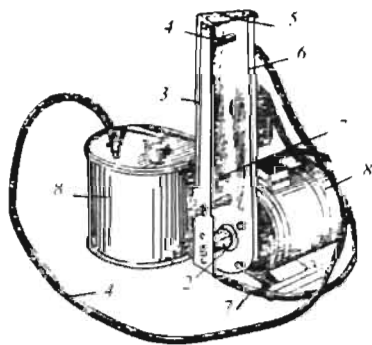
59-расм. Мумкатак рамкалардан асал олишда фойдаланиладиган титраб турадиган бугли пичок:
