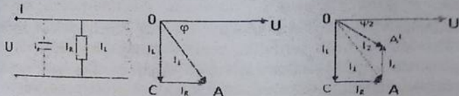
6.2-rasm. Reaktiv quvvatni kompensatsiyalash vektor diagrammasi.
