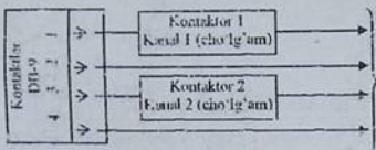
11.7-rasın. Yuklamani boshqarish zanjiriga ulash sxemasi
