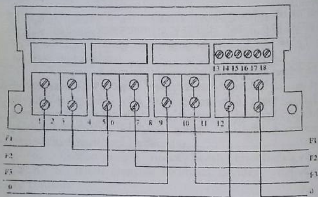
11.4-rasm. «Energiya – 9» CTK3-10A1HXR.VU hisoblagichi klemmlarining joylashishi
