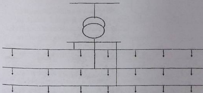
5.3-rasm. Shinali yig'malar bilan bajarilgan magistrall sxema.
