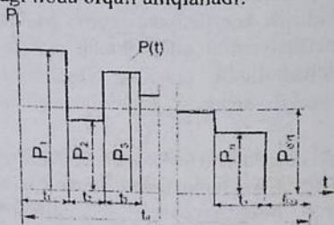
3.9-rasm. Yuklama grafigining vaqt boʻyicha notekisligi.
