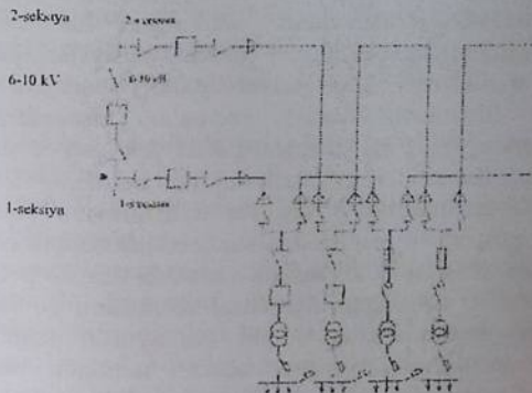
9.3-rasm. Ichki elektr ta'minoti sxemasi.
