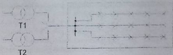
5.8-rasm. Sex yoritish tarmoqlarni ikki transformator yordamida ulash sxemasi.
