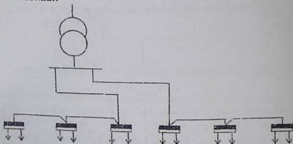
5.6-rasm. Aralash sxema.
