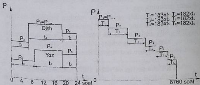
3.4-rasm. Yuklama davomiyligi bo'yicha yillik yuklama grafigi kurish usuli
