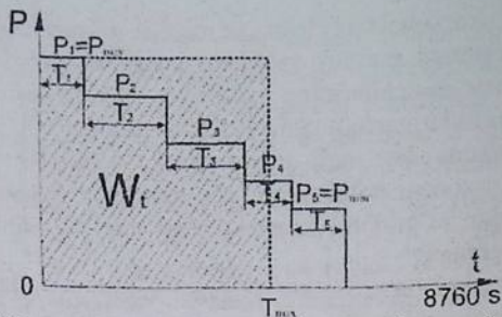
3.3-rasm. Davomiyligi bo'yicha yillik yuklama grafigi
