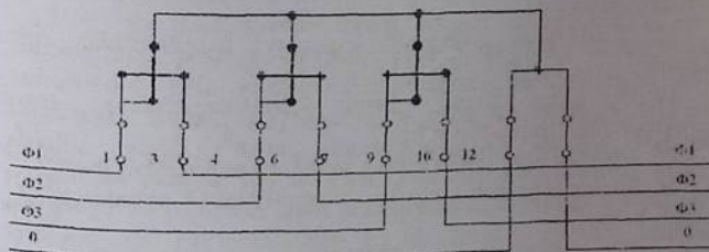
11.6-rasm. «Energiya -9» CTK3-10A1HXR.VU hisoblagichini
