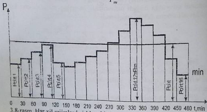
3.8-rasm. Har xil rejimlarda ishlovchi elektr iste'molchilarning yuklamalar grafiqi.
