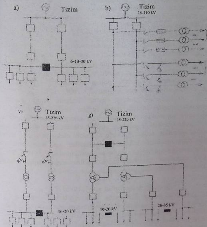
9.1-rasm. Tashqi elektr ta'minoti sxemalari.
