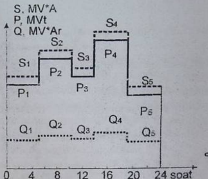
3.7-rasm. Iste'molchining aktiv, reaktiv va to'la quvvat bo'yicha sutkalik grafigi
