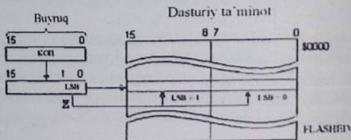
4.30-chizma. Konstantani adreslash
