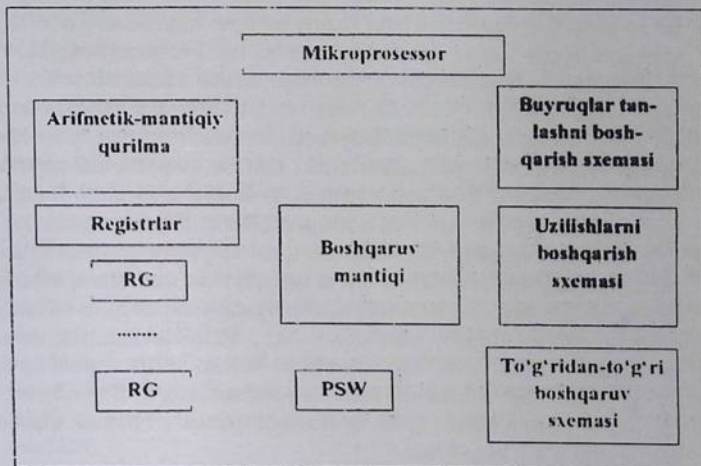
2.4-chizma. Oddiy MP ning tuzilishi
