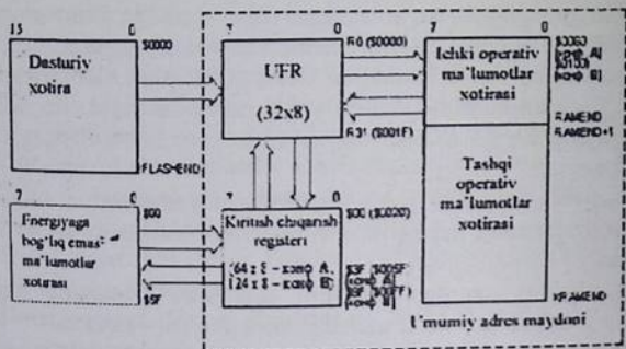
4.13-chizma. AVR-mikrokontrollerlarining dasturiy modeli
