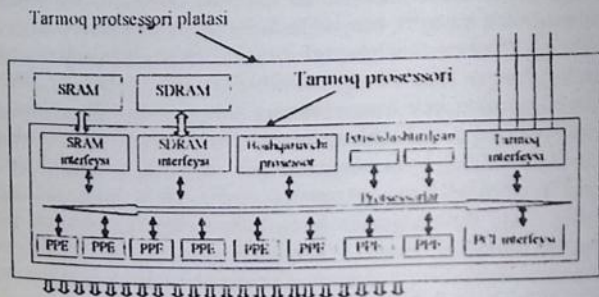
3.1-chizma. Odatiy tarmoq protsessorining kristali va platasi
