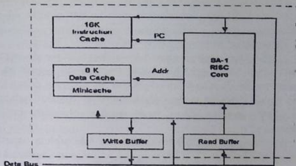
3.4-chizma. StrongARM mikroprotssori blok-sxemasi
