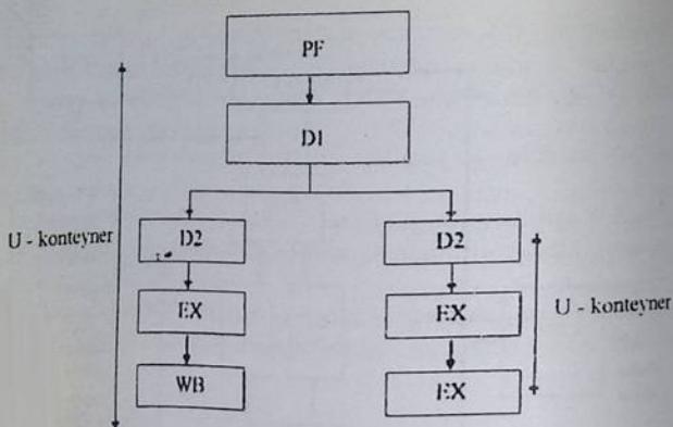
2.6-chizma. Pentium protsessorida butun sonli buyruqlarni bajarish bosqichlari
