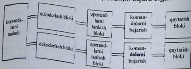
1.10-chizma. Komandalarni chaqiruvchi umumiy bo'limga ega besh bosqichdan iborat ikkitalik konveyer
