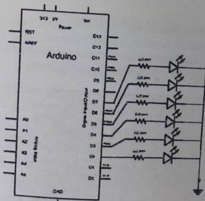
5.43-chizma. Arduino ga ulangan qurilmalarni boshqarish prinsipial sxemasi
