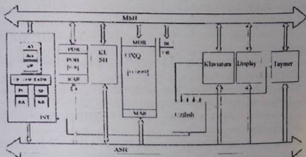
5.1-chizma. EHM o'quv modelining strukturaviy sxemasi
