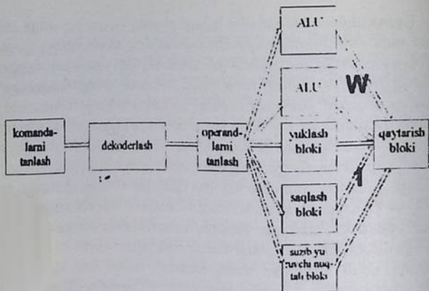
1.11-chizma. Beshta funksional bloklarga ega superskalyar protsessor
