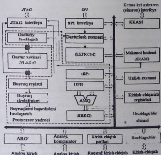
4.12-chizma. AVR oilasiga mansub mikrokontrollerlarning strukturasi
