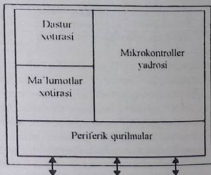
4.2-chizma. Mikrokontrollarning umumlashtirilgan tuzilmaviy sxemasi
