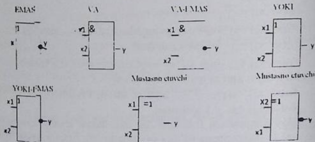
1.2-chizma. Mantiqiy elementlarning shartli belgilanishlari
