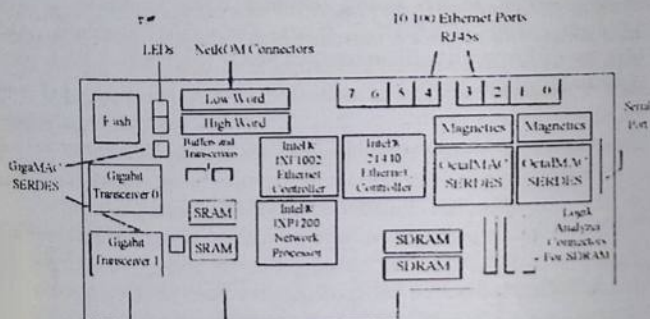
3.13-chizma. IXP1200 Ethernet Evaluation Board elementlari
