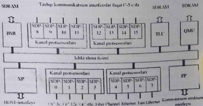
3.14-chizma. C-port turkumidagi tarmoq protsessorlarining umumlashtirilgan strukturasi
