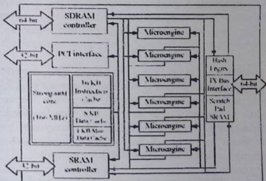
3.5-chizma. IXP1200 mikroprotssori blok-sxemasi
