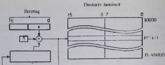
4.29-chizma. Dastur xotirasini nisbatan adreslash
