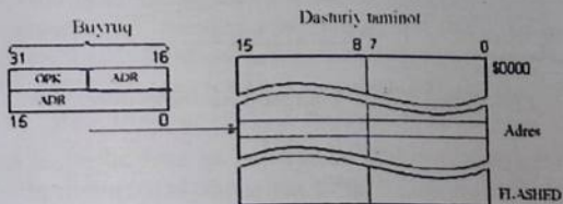
4.27-chizma. Dastur xotirasini bevosita adreslash
