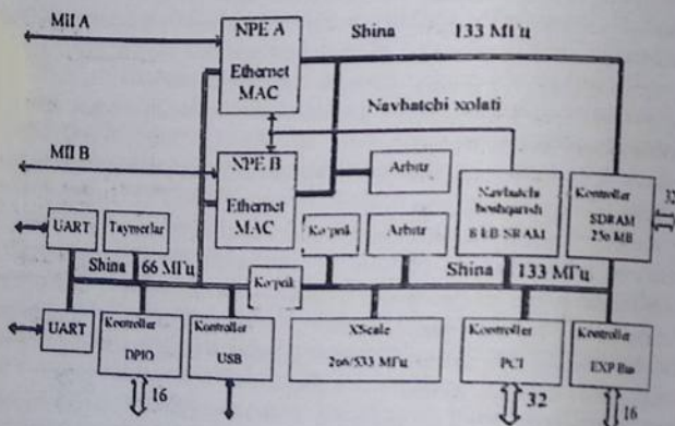
3.10-chizma. IXP420 protsessor arxitekturasida
