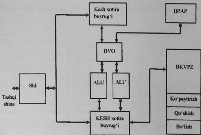
2.5-chizma. Pentium mikroprotssessorining umumlashgan struktura sxemasi
