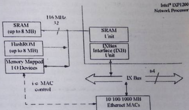
3.8-chizma. SRAM moduli, tashqi interfeyslar
