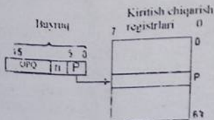
4.21-chizma. Kiritish-chiqarish registrini to'g'ridan-to'g'ri registrli adreslash
