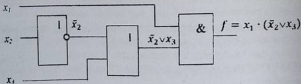
1.7-chizma. f = x_1 \cdot (\bar{x}_2 \vee x_3) funksiyaning kombinatsion sxemasi
