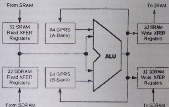
3.6-chizma. Registrlardan foydalanish
