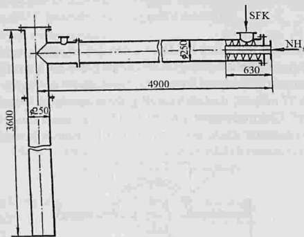
5.13- rasm. SFKni ammoniylash uchun quvurli reaktor sxemasi.
