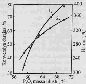
5.5- rasm. SKO'dagi P_2O_5 konversiya darajasi (1) va ammoniyashtirish harorati (2) ning boshlang'ich kislotaning konsentratsiyasiga bog'liqligi.
