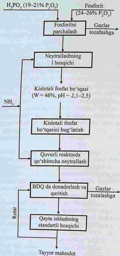
3.13-rasm. Ammofosfat ishlab chiqarish blok-sxemasi
