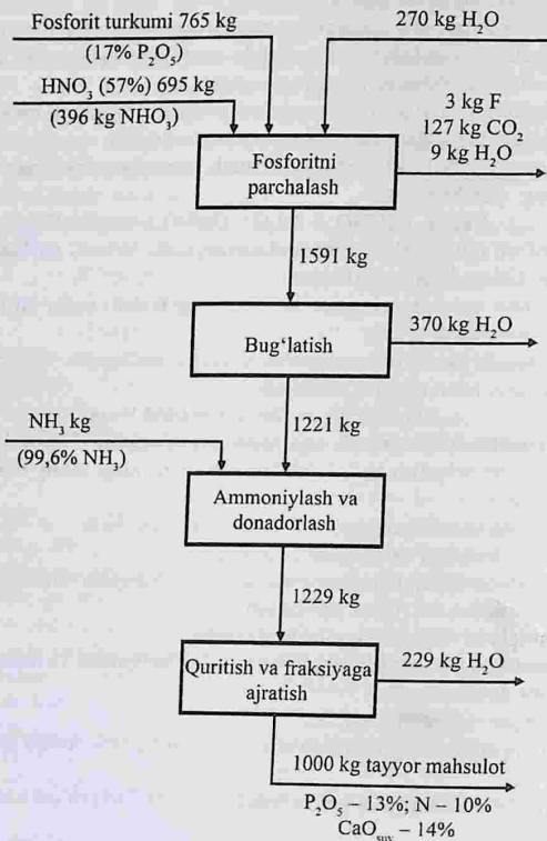
3.22- rasm. Nitrokalsiyfosfat ishlab chiqarish moddiy balansi.
