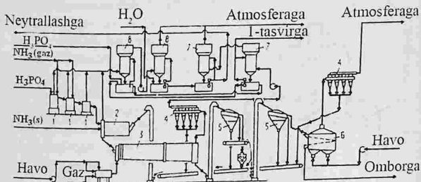
3.10- rasm. AD jihozi bilan donadorlangan ammosfos olish sxemasi:
