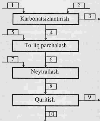
3.25-rasm. «PS-Agro» o'g'iti ishlab chiqarish moddiy balans sxemasi.
