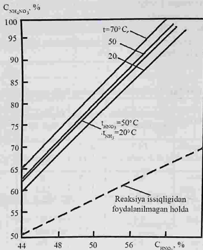
4.3- rasm. Reaksiya issiqligidan foydalanilganda olinadigan \text{NH}_4\text{NO}_3 eritmasi konsentratsiyasining reagentlar harorati turlicha bo'lganda nitrat kislota konsentratsiyasiga bog'liqligi (issiqlik yo'qotilishi 3% atrofida deb olinadi).
