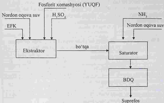
3.20- rasm. Markaziy Qizilqumni yuvib quritilgan fosforit konsratidan suprefos o'g'iti ishlab chiqarishning prinsipial texnologik sxemasi.
