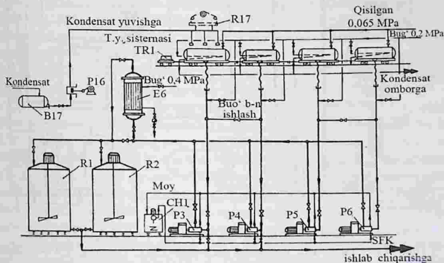
5.7- rasm. SFK qabul qilish va saqlash tarmog'i texnologik sxemasi:
