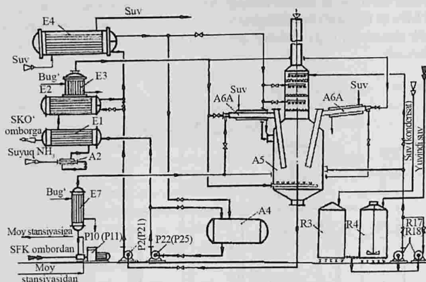
5.8- rasm. SKO' eritmasi olish tarmog'i texnologik sxemasi:
