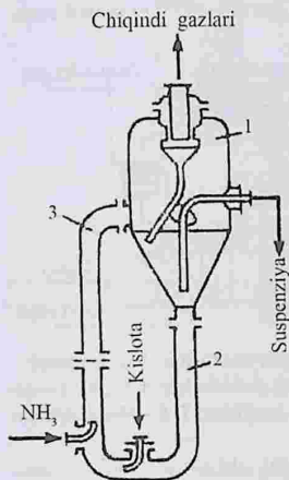
3.9- rasm. Tezkor ammoniy- lashtiruvchi bug'latgich (TAB).
