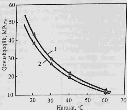
5.2- rasm. SKO' qovushqoqligining haroratga bog'liqligi.
