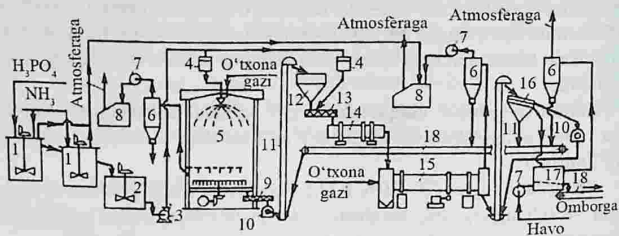
3.6- rasm. Changlatgichli quritgichda ammosfos ishlab chiqarish sxemasi:
