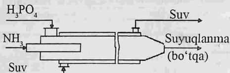
3.16- rasm. Tezkor oqimli reaktor.
