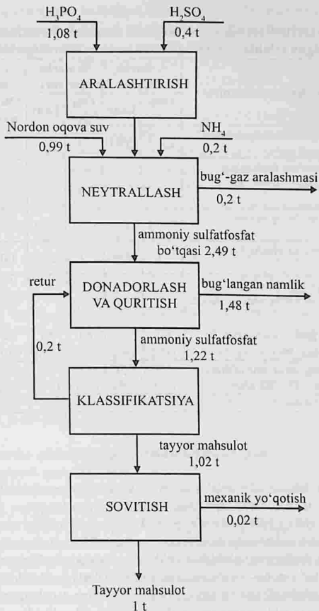
3.18- rasm. A navli ammoniy sulfatfosfat o'g'itining olish moddiy balansi.
