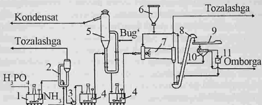
4.7- rasm. Karboammofos olish texnologik sxemasi:
