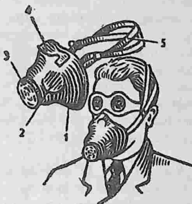
4-rasm. Resperator R-2: 1-yarim niqob; 2-nafas olish klapani; 3-nafas chiqarish klapani; 4-burun qisqichi; 5-tasmalar
