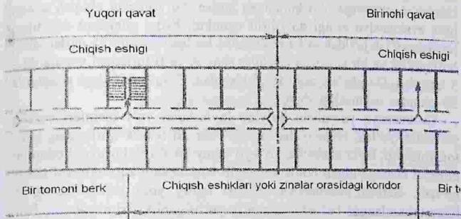
7-rasm. Evakuatsiya yo'llarining tarkibiy qismlari
