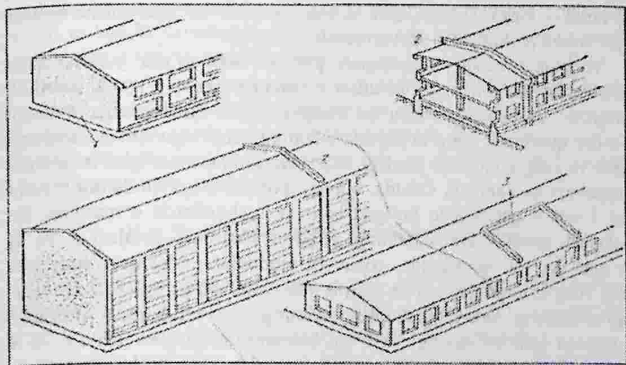
8-rasm. Binolarda yong'inga qarshi devorlarning o'rnatilishi:
