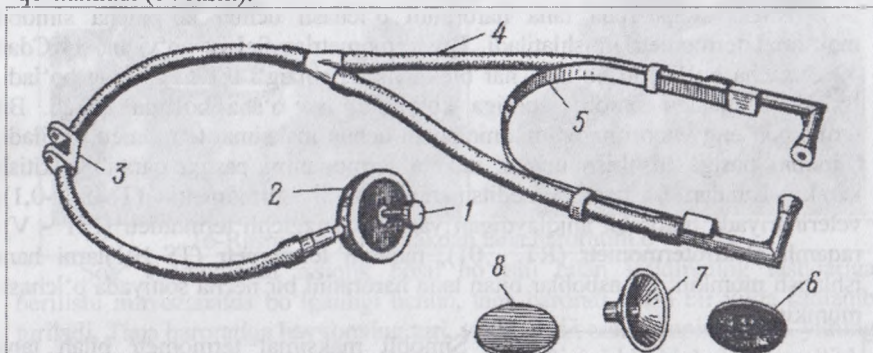
14-Rasm. Stetofonendoskop: 1-pelot, 2-fonendoskop bosh qismi, 3-pelot ushlagichi, 4-egiluvchan tovush o'tkazgich, 5-metall ushlagich, 6-membrana, 7-stetoskop rupori, 8-fonendoskop bosh qismi qopqog'i
