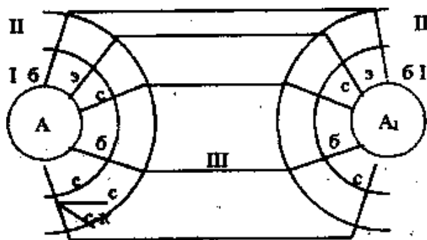
Рис. 3. Схема конвергенции энергетических связей. А (автотроф), I, П – концентры; б – биотрофные связи, с – сапротрофные, э – экрисотрофные, с-к – копротрофные (сапротрофные) связи.
