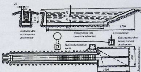
Рис. 170. План ванны для купания овец
