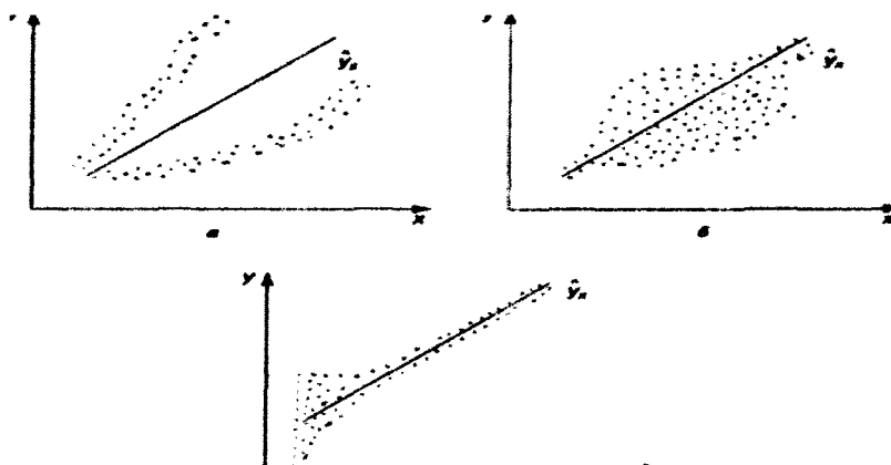
5.1.-rasm. Geteroskedatlik holatlari 3
