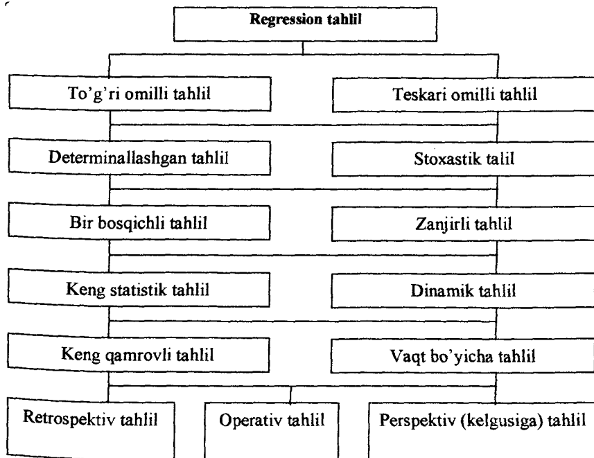
3.1-rasm. Regression tahlilning masalalar tavsifining umumlashgan sxemasi
