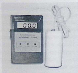
Рисунок 2. Газоанализатор ХОВВИТ-Т, измеряющий количество и качество газов
