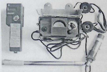
7- Изображение. Обзор радиометра ДП-5В (А) и дозиметра ИПД-02Б 16 (Б)
