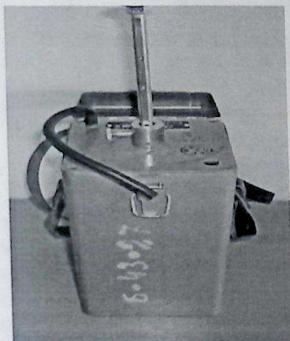
Рисунок 3. Газоанализатор УГ-2
