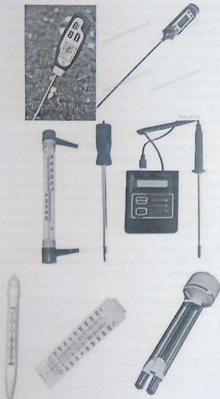
Рисунок 11. Термометры и психрометры разных моделей, измеряющие температуру помещения, воды и почвы.
