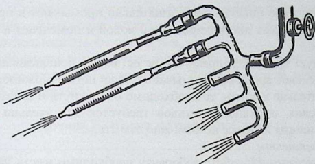
Рисунок 92 – Приспособление для промывания пипеток
