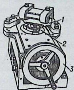
Рисунок 100 — Ротационный микротом для резки объектов без декальцинации: 1 — нож; 2 — объектодержатель; 3 — устройство для движения каретки с объектодержателем
