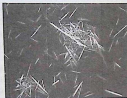
Рисунок 79 – Кристаллы урата натрия: поляризационная микроскопия
