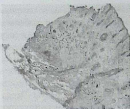
Рисунок 140 – Фрагмент кожных покровов и подкожной клетчатки (окраска гематоксилином Эрлиха и эозином)
