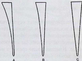
Рисунок 105 – Типы микротомных ножей (А, В, С)
