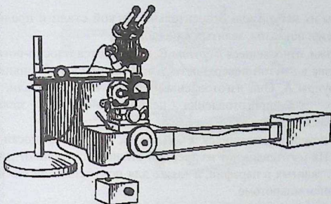
Рисунок 104 – Ультрамикротом тепловой УМТ-2
