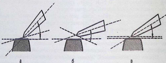
Рисунок 132 – Угол наклона микротомного ножа: а – слишком большой; б – слишком маленький; в – правильный ( 15^\circ )
