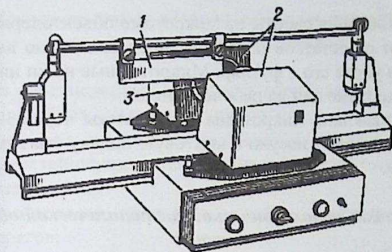
Рисунок 106 – Станок для заточки микротомных ножей ЗМН-2:
