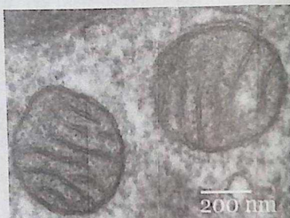
Рисунок 87 – Митохондрии: просвечивающая электронная микроскопия
