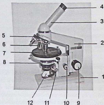
Рисунок 73 – Устройство светового микроскопа: 1 – основание микроскопа; 2 – тубусодержатель; 3 – тубус; 4 – окуляр (чаще \times 7 ); 5 – револьвер микроскопа; 6 – объективы (а – сухие: \times 8 , \times 20 , \times 40 ; б – иммерсионный \times 90 ); 7 – предметный столик; 8 – конденсор; 9 – макрометрический винт; 10 – микрометрический винт; 11 – винт конденсора; 12 – зеркало
