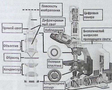
Рисунок 78 – Конфигурация фазово-контрастного микроскопа
