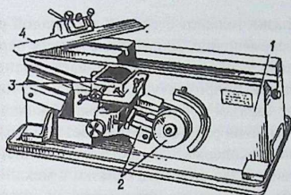
Рисунок 94 – Саный микротом: 1 – станина микротомы; 2 – устройство, поднимающее объект на заданную высоту; 3 – объектодержатель; 4 – нож, закрепленный в «салазках», скользящих по направляющим станины
