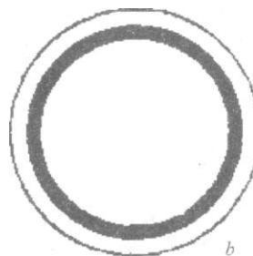
40- rasm. Fazo-kontrast qurilmasini sozlashda yordamchi mikroskopning kuzatish mavdonidagi halqalarning holati: a - noto'g'ri; b - to'g'ri.
