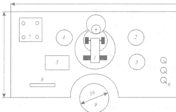
41- rasm. Mikroskop bilan ishlashda tekshiruvchining ish joyini tashkil qilish sxemasi.
