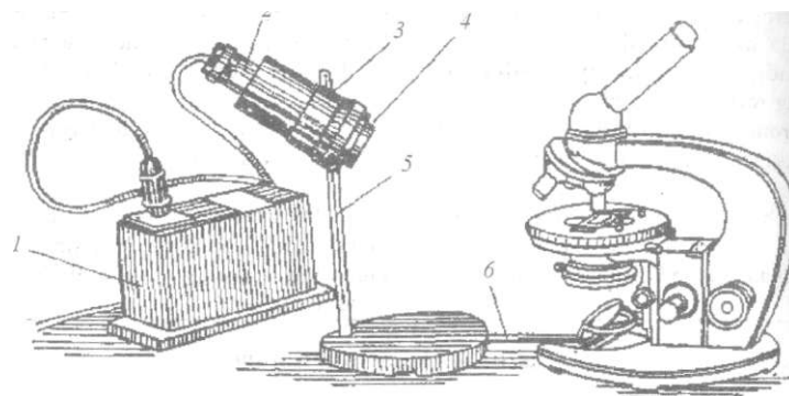
39- rasm. Fazo-kontrast qurilmasi:
