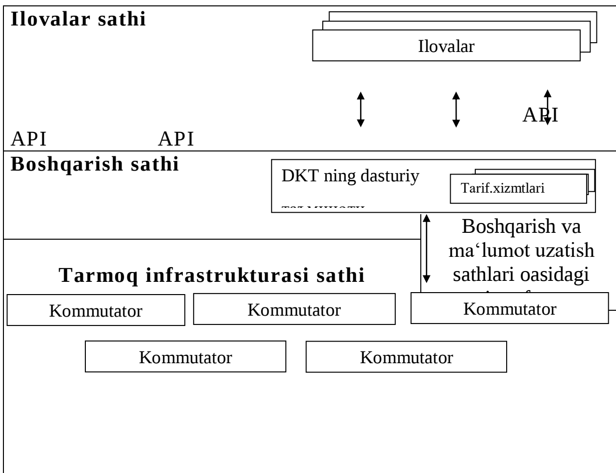
3.3 – rasm. Dasturiy konfiguratsiyalanadigan tarmoq arxitekturası.
