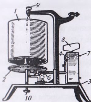
37-rasm. Kimograf: 1-baraban, 2-disk, 3-shtativ va unga o'rnatilgan 4 – sout mexanizmi, 5 – muffa, 6 – asos yoki o'q, 7 – uzatgich, 8 – flyuger, 9 – yuqori va 10 – pastki vint
