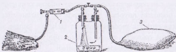
20-rasm. Itga efir-kislorod narkoz berish asbobi: 1-nafas olish va nafas chiqarish uchun jo‘mrak; 2-vul‘fning ikki og‘izli shisha idishi; 3-kislorodli yostiq
