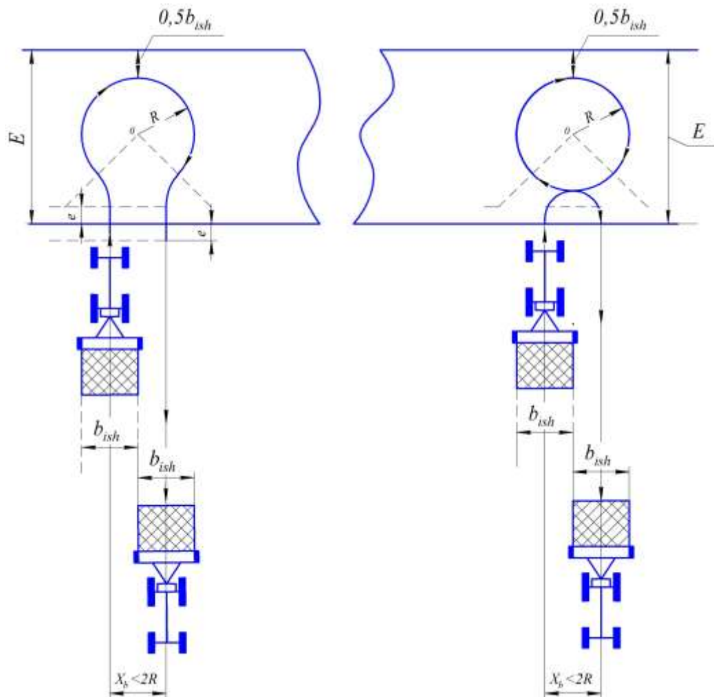
17-rasm. Sirtmoqli burilish joyida agregatlarning parakatlanish troektoriyasi
