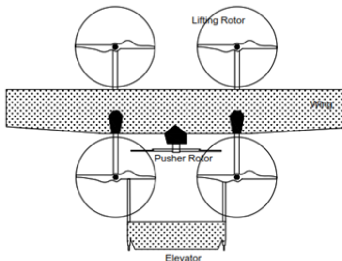
10.9-rasm. Gibrid uchish jixoziga ega uchuvchisiz uchish vositasi konstruktsiyasi
