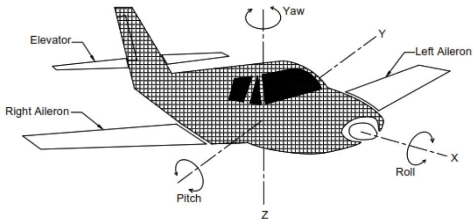
10.7-rasm. Qo'zg'almas qanotli uchuvchisiz uchish vositasi konstruktsiyasi
