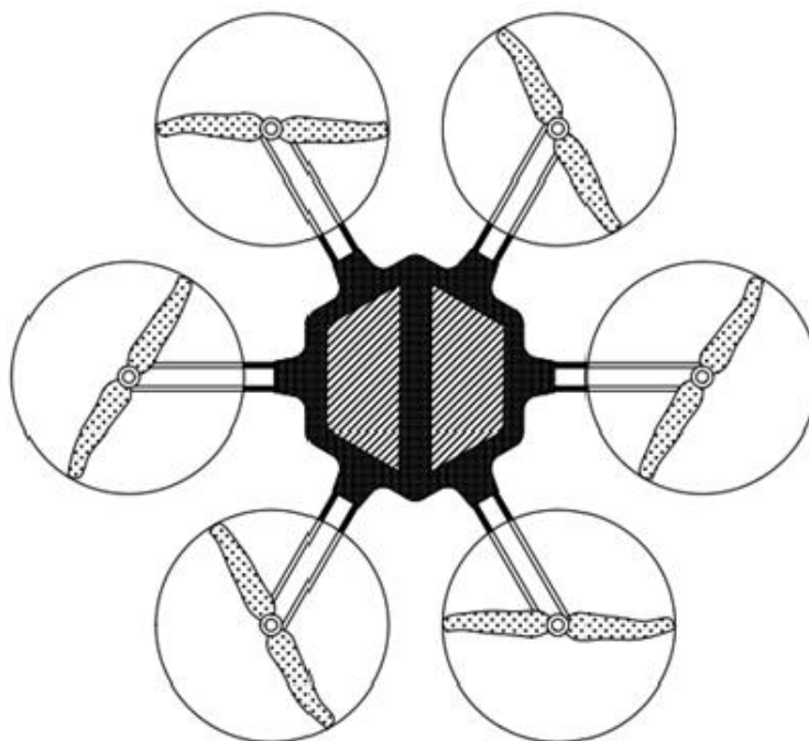
10.12-rasm. Hexacopterlarning konstruktsiyasi
