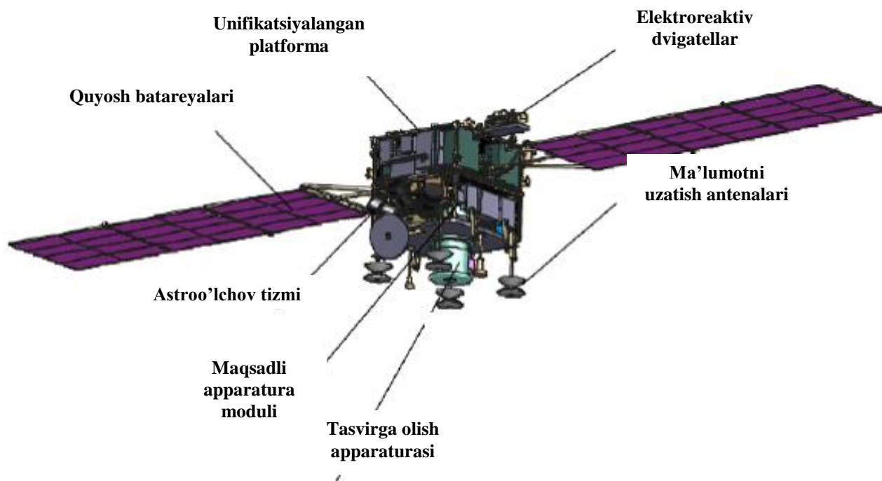
4.4-rasm. Masofadan zondlashda foydalaniladigan sun'iy yo'ldoshlarning umumiy ko'rinishi
