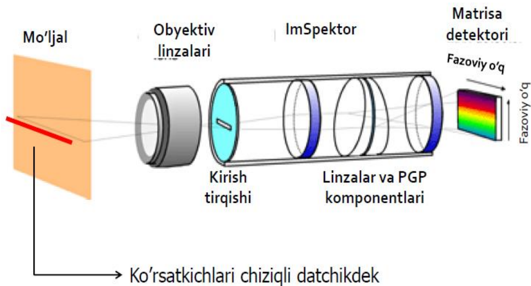
5.8-rasm. Optik kamera tuzilishi va ishlash prinsipi
