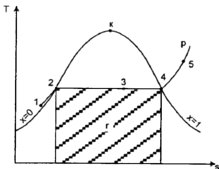
2.1-rasm. Suv bug'ining fazaviy T, s - diagrammasi
