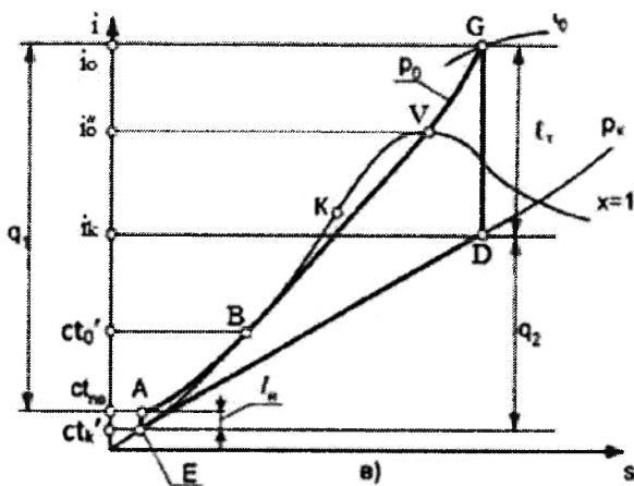
1.13-rasm. Bug'ni ortiqcha qizitish bilan kechadigan Renkin sikli
