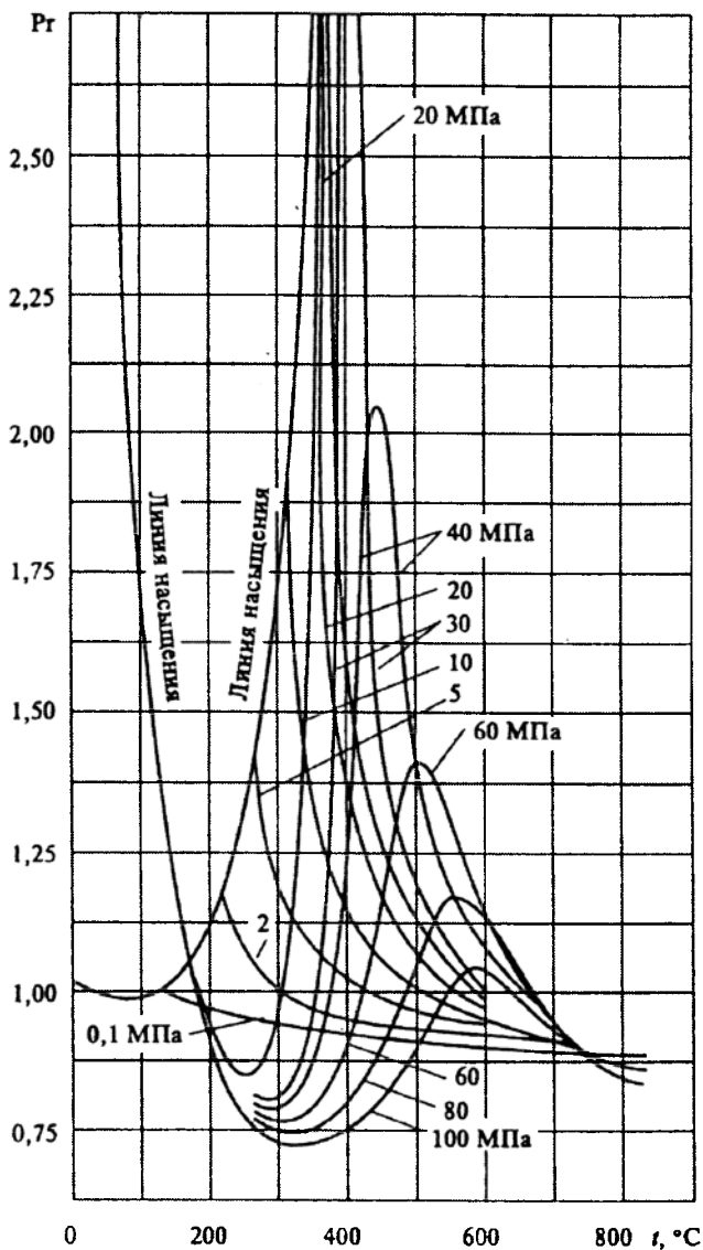
5-рasm. Prandtl suv va suv bug'i miqdorini harorat va bosimga bog'liqligi
