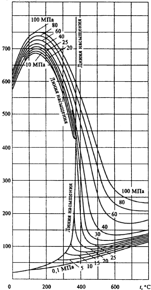
4-рasm. Suv va suv bug' issiqlik va bosimning issiqlik o'tkazuvchanligiga bog'liqligi
