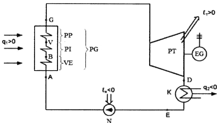
1.12-rasm. Bug‘-kuch uskunasiining prinsipial sxemasi:
