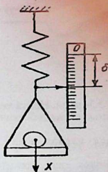
32. расм. Бевосита баҳолаш усули
