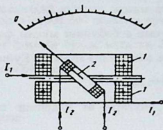
5.4-расм. Электродинамик ўлчаш асбоби
