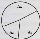
4.1-Ўлчаш хатоликлари.
