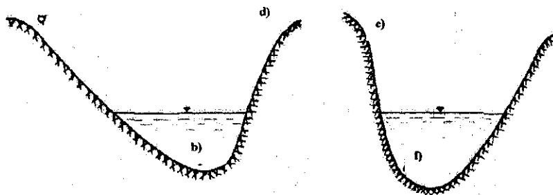
5.3-rasm. B. Daryo qirg'og'ining turlari
