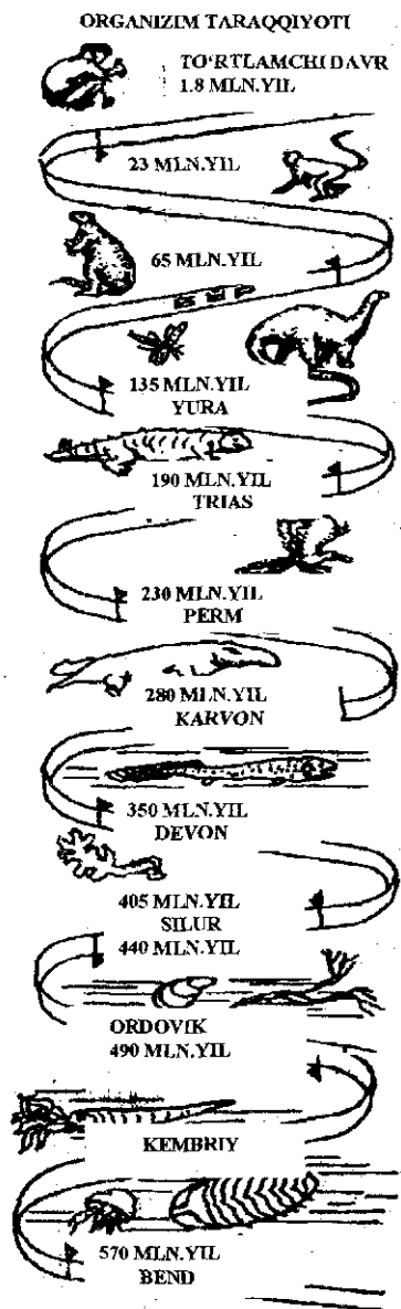
2.1-rasm. Geoxronologik shkalaning Kembriydan to'rtlamchi davrgacha tavsifi
