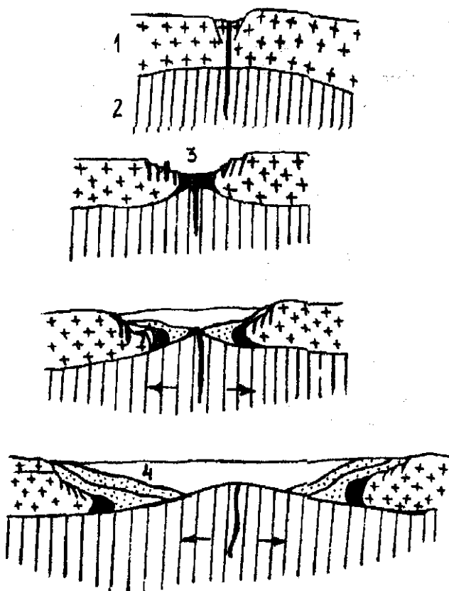
4.2-rasm. Chekka okean qismlaridagi harakatlar
