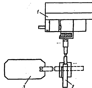
11.3- rasm Bir pozitsiyali robototexnik kompleks: 1-tokar dastgohi; 2-sanoat roboti; 3-gorizontal magazin to'plagich.
