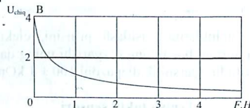
10.3- rasm. Elastomer taktill sensorning chiqish xarakteristikalari.
