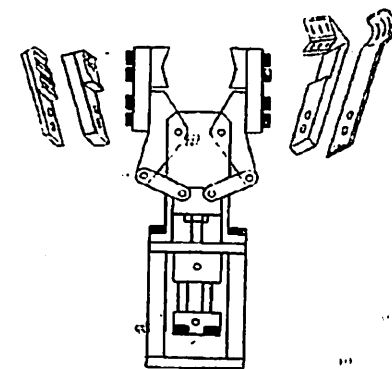
2.14 - rasm. Richagli qisqich qurilmasi.
