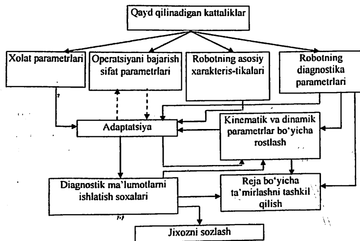
12.5. - rasm. Robotning nazorat qilinadigan asosiy parametrlarining strukturasi.
