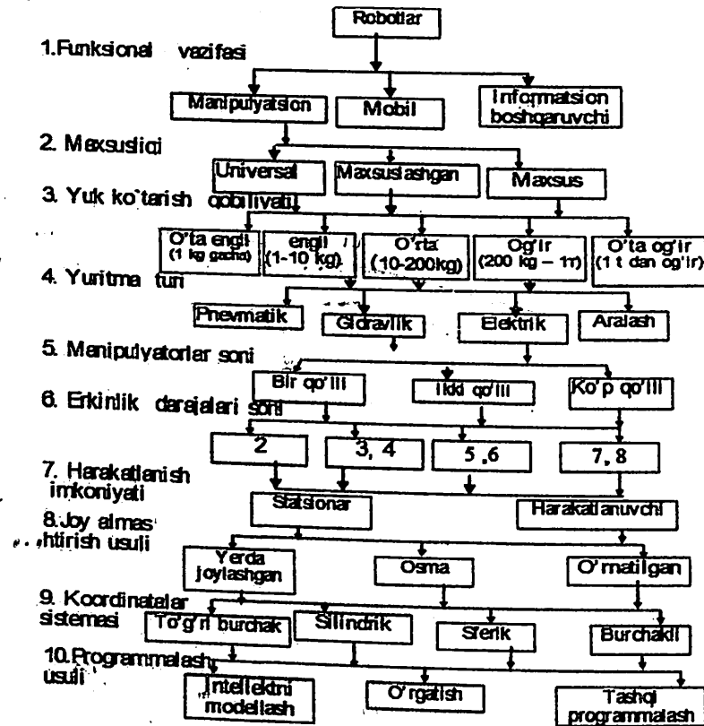
1.1- rasm. Sanoat robotlarining sinflanishi
