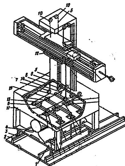
3.8- rasm. Ko‘p koordinatali yuritmalı sanoat robotining konstruktiv sxemasi:
