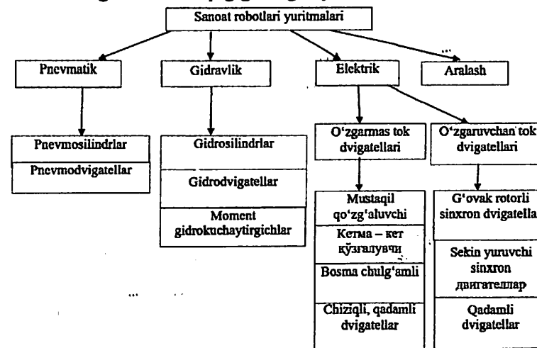
3.1 – rasm. Sanoat robotlari yuritmalarining sinflanishi.
