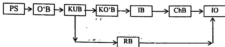
4.7 - rasm. Sanoat roboti kontur boshqarish qurilmasining struktura sxemasi:
