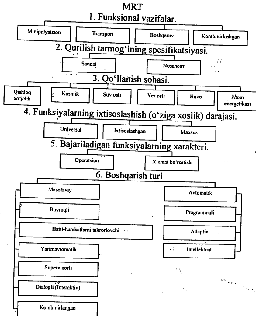
9.2 - rasm. MRT larning umumlashgan alomatlariga ko'ra sinflanishi.
