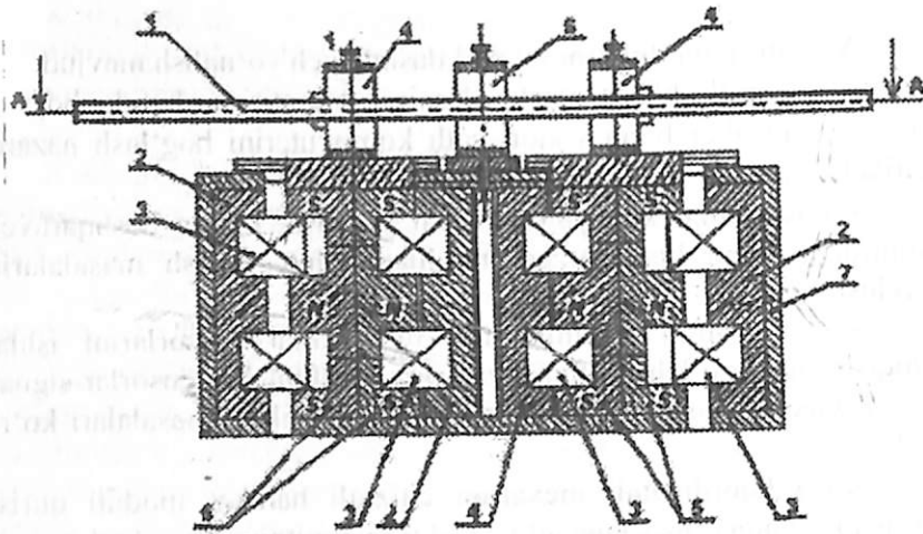
15.4-rasm. Bir-biriga bog'liq bo'lmagan uchta chiziqli ko'p koordinatali KMHning konstruksiyasi:
