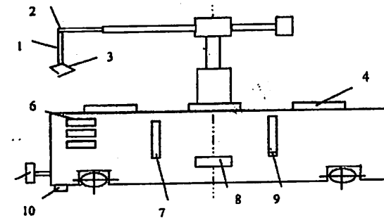
9.3-rasm. MP-12t robokarasida tashqi informatsiya datchiklarining joylashtirilishi:
