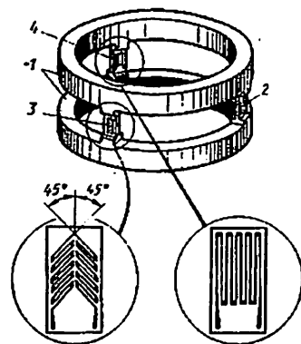
10.6- rasm. Kuch va moment datchigi:
