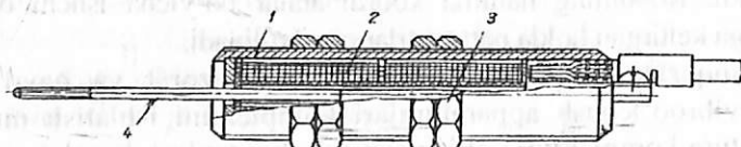
12.1-rasm. Induktiv siljish datchigining konstruksiyasi
