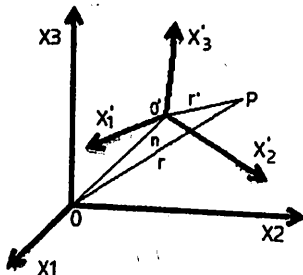
2.13-rasm. Manipulyator koodinat tizimi.
