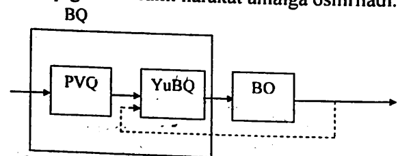
4.1 - rasm. Sanoat roboti boshqarish tizimining funksional sxemasi: BQ - boshqarish qurilmasi; PVQ - programma - vaqt qurilmasi; YuBQ - yuritmalarni boshqarish bloki; BO - boshqarish ob'yekti (sanoat robotining ishchi qurilmalari).
