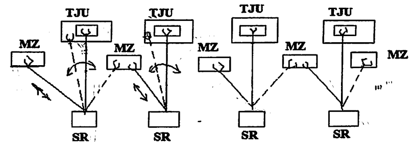
6.11 - rasm. RTK ning chiziqli joylashtirilish sxemasini: MZ-xom mahsulotni dozalab berib turuvchi magazin.
