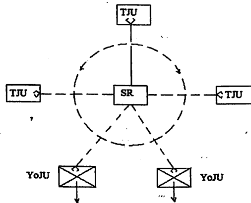
6.9 - rasm. Guruhli RTK lar.
