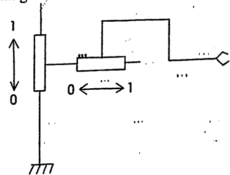
13.9 – rasm. Manipulyatorning kinematik sxemasi.
