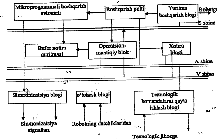
4.6- rasm. Unifikatsiyalangan pozitsion programmani UPM-772 tipidagi boshqarish qurilmasining struktura sxemasi.
