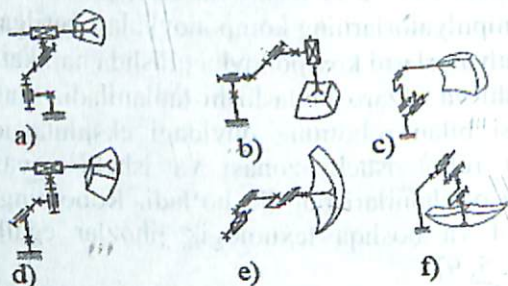
2.10– rasm. Sferik koordinatalar sistemasidagi kinematik sxemalar.
