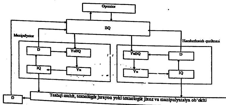
1.2 - rasm. Sanoat robotining struktura sxemasi: BQ - boshqarish qurilmasi, YuBQ - yuritmalarni boshqarish qurilmasi; D - datchik; Yu - yuritma; ishchi qurilmasi.
