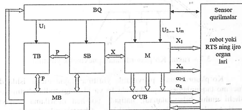
3.6 - rasm. Ko'pkoordinatali yuritmaning umumlashgan struktura sxemasi.
