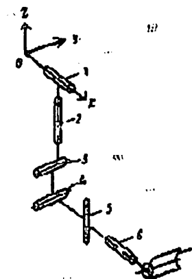
2.2 – rasm. Robot qo'li mexanizmining sxemasi: 1,2,3-regional harakatlar; 4,5,6- orienterlash harakatlari; 7- ishchi organ;
