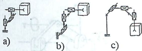
2.8– rasm. To‘g‘ri burchak koordinatalar sistemasida ishlovchi manipulyatorlarning kinematik sxemalari:
