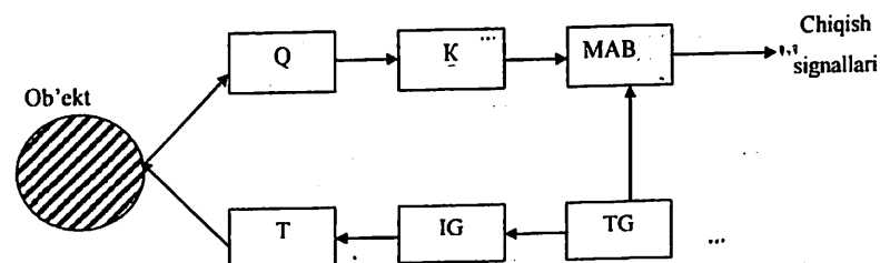
10.5- rasm. Lokatsion datchikning struktura sxemasi: Q- qabul qiluvchi qurilma; K- kuchaytirgich; MAB- masofani aniqlash blogi; T- to'lqin tarqatuvchi qurilma; IG- impuls generatori; TG-tayanch generatori.
