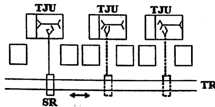
6.12 - rasm. Qo'zg'aluvchan robotli RTL sxemasi: QSR - qo'zg'aluvchan sanoat roboti, M - magazin, TR - Sanoat robotining harakat chizig'i (trassasi).
