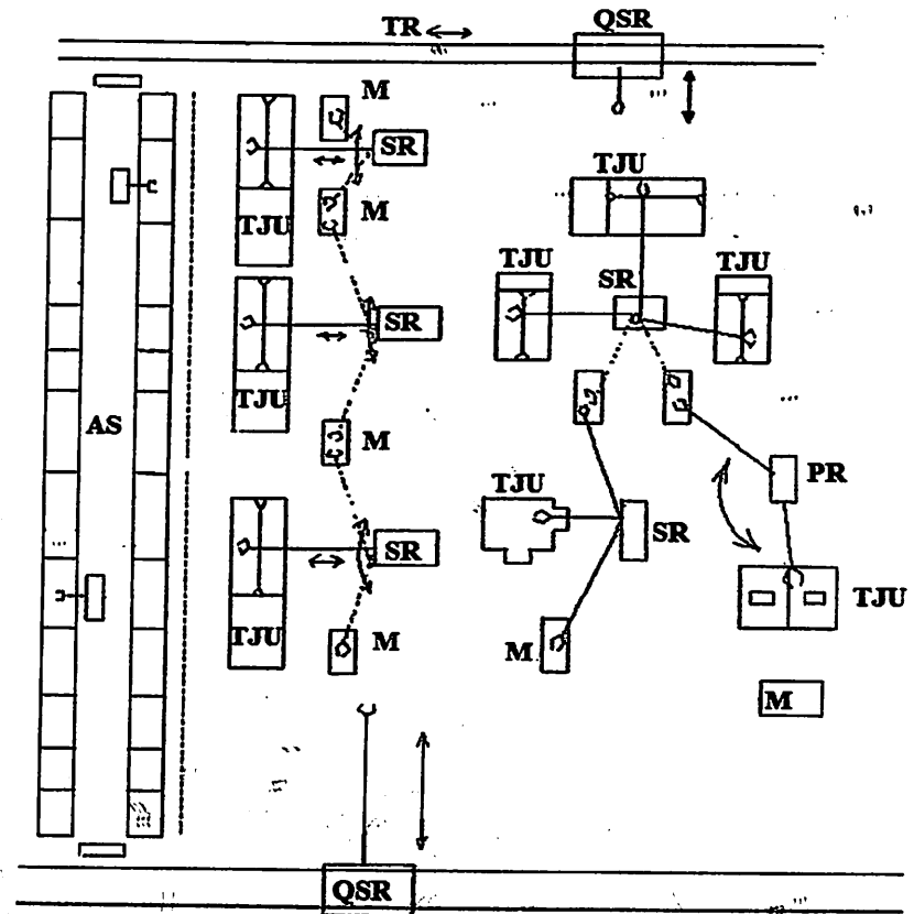
6.14 - rasm. Robotlashtirilgan texnologik kompleksning chiziqli aylanali joylashtirish sxemasi.
