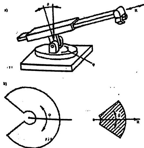
2.6 -rasm. Sferik koordinatalar sistemasidagi robot va uning ishchi zonasi: a) robotning konstruktiv sxemasi, b) ishchi zonasi
