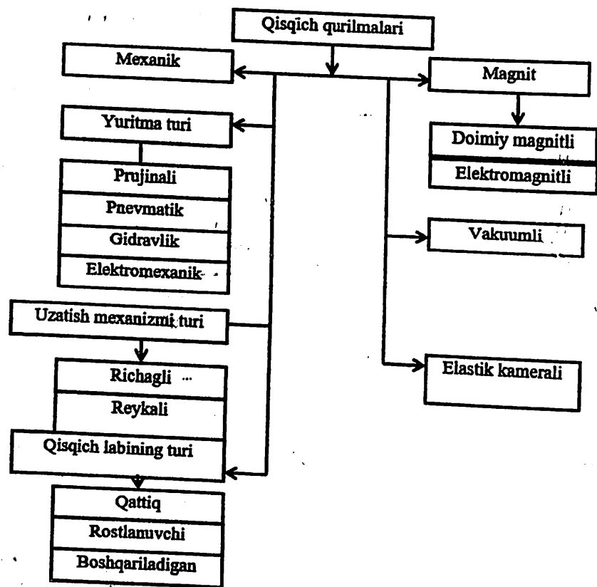
2.13 - rasm. Qisqich qurilmalarining sinflanishi.
