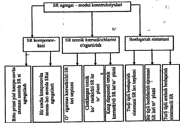
1.6 – rasm. Sanoat robotlarini agregat – modul qurishning struktura sxemasi.
