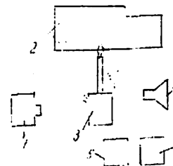
8.1 - rasm. Robotlashtirilgan ishchi pozitsiya sxemasi: 1-uzatib turuvchi qurilma; 2 - stanok; 3 - sanoat roboti; 4-olib turuvchi qurilma; 5- SRning boshqarish qurilmasi; 6 - dastgoh (stanok)ni boshqarish qurilmasi.
