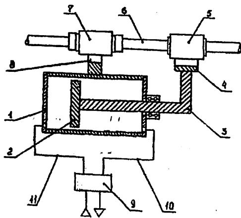
3.7 – rasm. Ko‘pkoordinatali pnevmatik yuritma.
