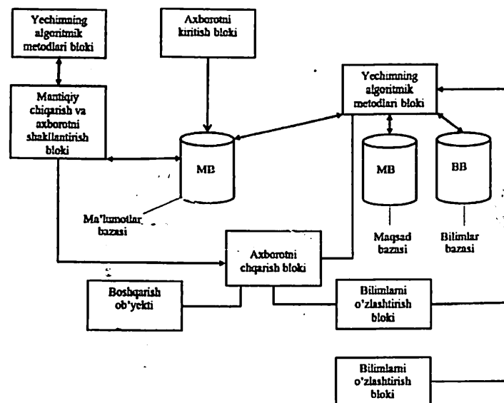
13.5-rasm. Intellektual robototexnik tizimning struktura sxemasi
