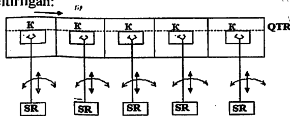
6.13-rasm. Yig'uv RTL ning chiziqli joylashtirish sxemasi: QTR - qadamlı transportyor; K - kassetalar.
