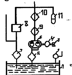
3.4 – rasm. Sanoat roboti gidrostansiyasining funksional sxemasi
