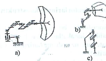
2.11 – rasm. Burchak koordinatalar sistemasidagi kinematik sxemalar.
