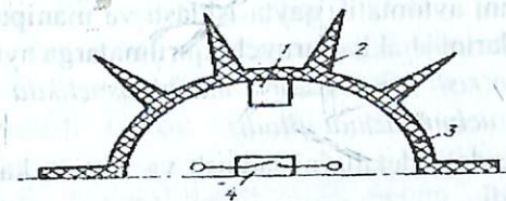
10.2- rasm. Taktil tegish sensori:
