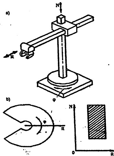
2.5 rasm. Silindrik koordinatalar sistemasida ishlovchi robot va uning ishchi zonasi: a) robotning konstruktiv sxemasi, b) ishchi zonasi
