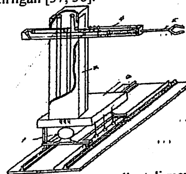
15.5- rasm. Ko'p koordinatali mexatron modul asosida qurilgan sanoat roboti
