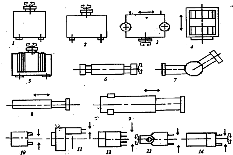
1.7 – rasm. Robot manipulyatorining unifikatsiyalangan modullari: 1 – ko'tarish va burilish moduli; 2 – burilish moduli; 3 – burilish va siljish moduli; 4 – ko'tarish moduli; 5 – burilish va chiziqli harakat moduli; 6 – aylanish moduli; 7 – tebranma harakat moduli; 8 – siljish moduli; 10 – 14 qisqich modullari.
