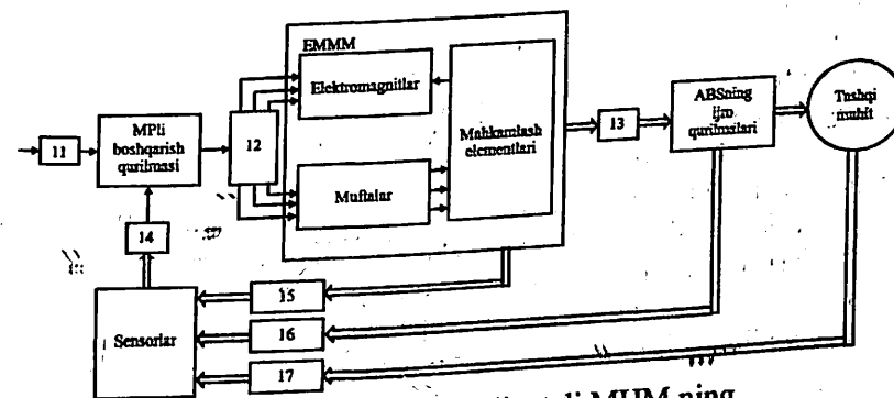
15.3-rasm. Ko'p koordinatali MHM ning umumlashgan struktura sxemasi
