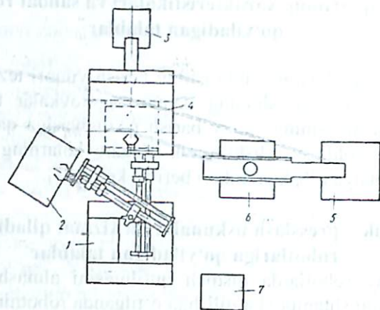
11.1- rasm. Pressga xizmat eiluvchi robot asosidagi robototexnik kompleks
