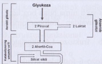
Glyukoza katabolizmining sxemasi
