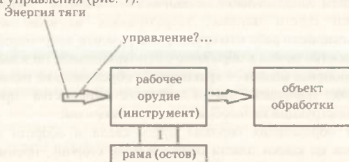
Рис. 7 Начальное структурирование сельскохозяйственного орудия — конного плуга
