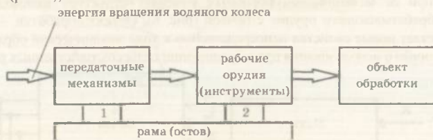
Рис. 8 Структурная схема элементарной технической системы природным источником механической энергии
