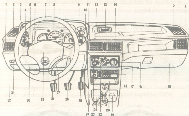
5-rasm. «Neksiya» avtomobilidagi boshqaruv jihozlarining joylashuvi:
