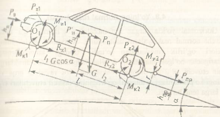
28-rasm. Balandlikka chiqayotgan avtomobilga tezlanish vaqtida ta'sir etayotgan kuchlar.
