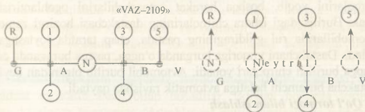
9-rasm. «VAZ – 2109» avtomobilining uzatmalarini qo'shish sxemasi:
