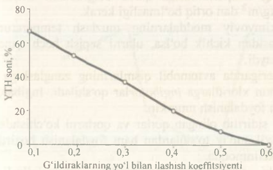
50-rasm. G'ildiraklarning yo'l bilan ilashish koeffitsiyentini ( \phi ) YTH miqdoriga ta'sir grafigi.
