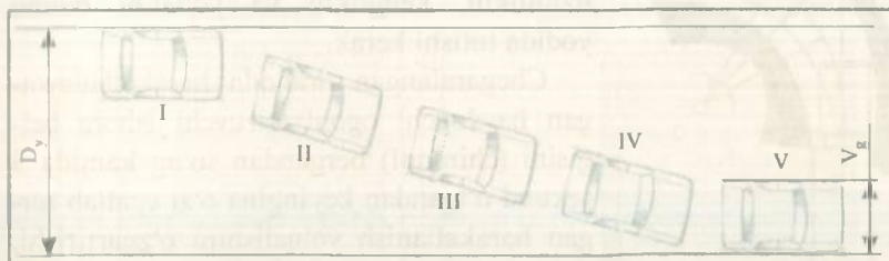
16-rasm. Yo'lining to'g'ri qismidagi avtomobilning dinamik yo'lagi:
