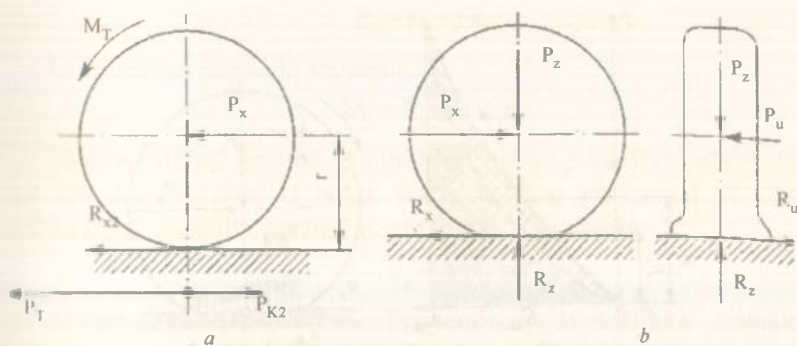
24-rasm. Yo'lning g'ildirakka ta'sir etuvchi reaksiyalari:
