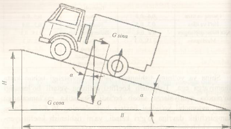
26-rasm. Avtomobilning balandlikka chiqishiga qarshilik kuchi.
