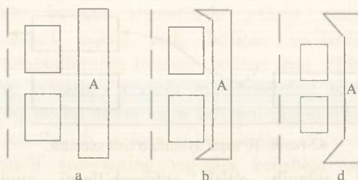
43-rasm. Avtobus bekatlarining turlari: a –yo'ning qatnov qismida joylashgan; b –yarim cho'ntak ko'rinishidagi; d –cho'ntak ko'rinishidagi bekatlar.
