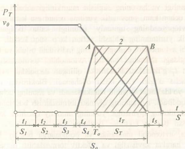
30-rasm. Avtomobilning tormozlanish protsessi grafigi.
