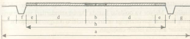
61-rasm. Ikki tasmani avtomobil yo'lining ko'ndalang kesimdagi ko'rinishi: a —yo'l poyi; b —ajratuvchi tasma; d —qatnov qismi; e —yo'l yoqasi; f —ariq; g —yo'l cheti; h —yo'l bo'lagi.
