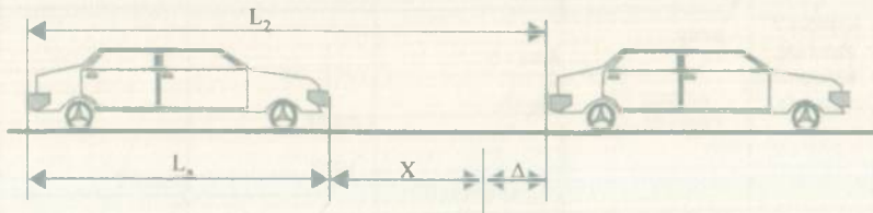
15-rasm. Avtomobilning dinamik gabarit uzunligi:
