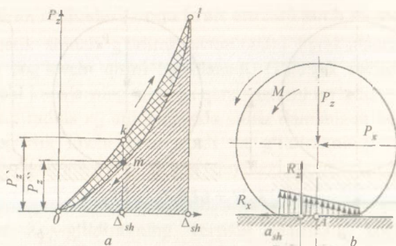
25-rasm. G'ildirashga qarshilik:
