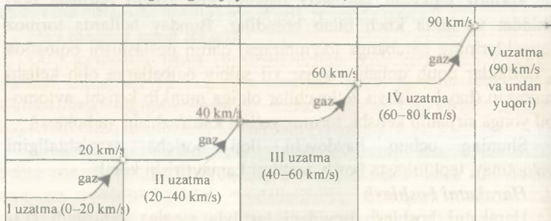
14-rasm. Uzatmalar qutisini yuqori pog'onalariga o'tkazish bosqichlari.
