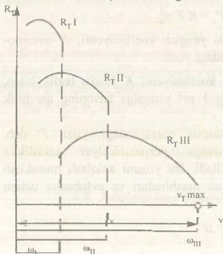
27-rasm. Avtomobilning tortish xarakteristikasi.
