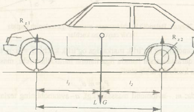
29-rasm. Harakatsiz avtomobilga ta'sir etuvchi kuchlar.
