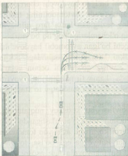
33-rasm. Avtomobilning o'ngga burilish sxemasi.
