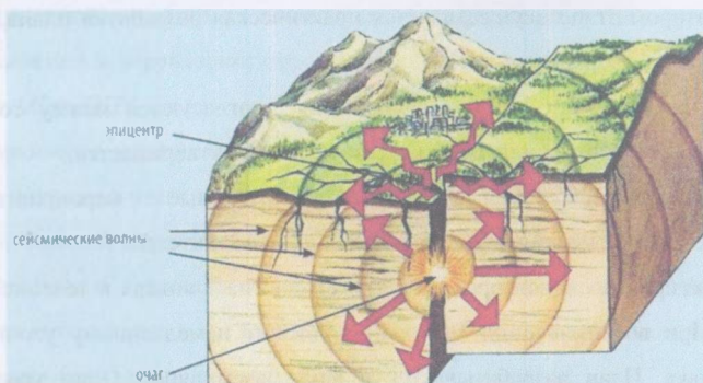
Рис. 3.14. Распространение сейсмических волн от центра землетрясения.
