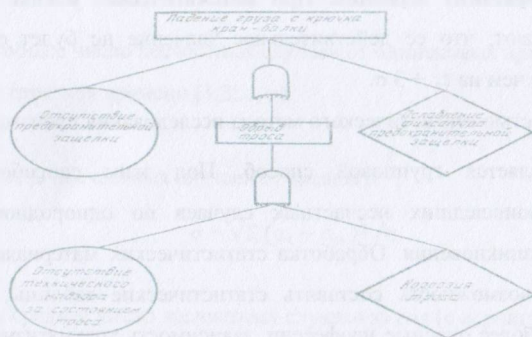
Рис. 2.2. Схема, построенная по методу «Дерево отказов»
