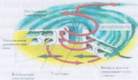
Рис. 3.9. Разрез урагана
