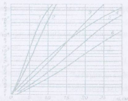
Рис. 2.10. Зависимость кратности ослабления \gamma -излучения от толщины защитного экрана:
