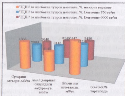
2-расм. Тажириба даласининг вариантлар буйича ўртача сув истеъмоли, 2015 й.
