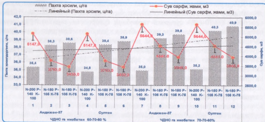
3-расм. Тажриба вариантлари бўйича олинган пахта ҳосилдорлиги ва сарфланган сув миқдорлари, 2015 й.
