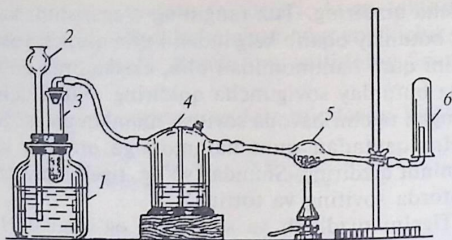
24-rasm. Oksid tarkibini aniqlash asbobi.
