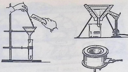
13-rasm. Issiq filtrlash uchun elektr toki va gaz bilan isitiladigan voronkalar.
