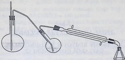
19-rasm. Suv bug'i bilan haydash asbobi.
