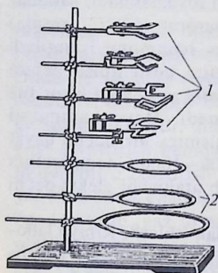
6-rasm. Laboratoriya shtativi: 1 — qisqichlar; 2 — tagliklar.
