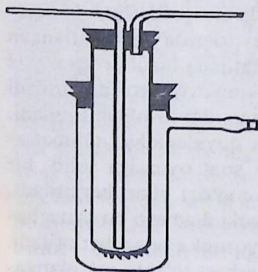
16-rasm. Vakuumda sublimatsiya qilish asbobi.
