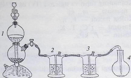
22-rasm. Uglerod (IV) oksidni olish va uni tozalash uchun qurilma: 1 — Kipp apparati; 2, 3 — Tishenko sklyankalari; 4 — yassi tubli kolba.
