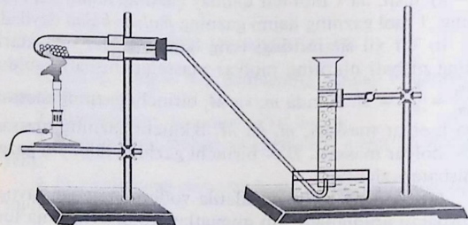
21-rasm. Tez uchuvchan moddalarning molekulyar massasini Meyer usulida aniqlash uchun ishlatiladigan asbob.
