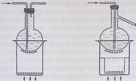
15-rasm. Moddalarni sublimatlash yo'li bilan tozalash.
