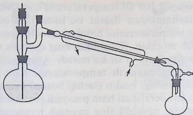
18-rasm. Vakuumda haydash asbobi.
