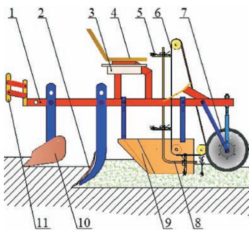
Рис. Конструктивная схема комбинированного почвообработавше-посадочного агрегата
