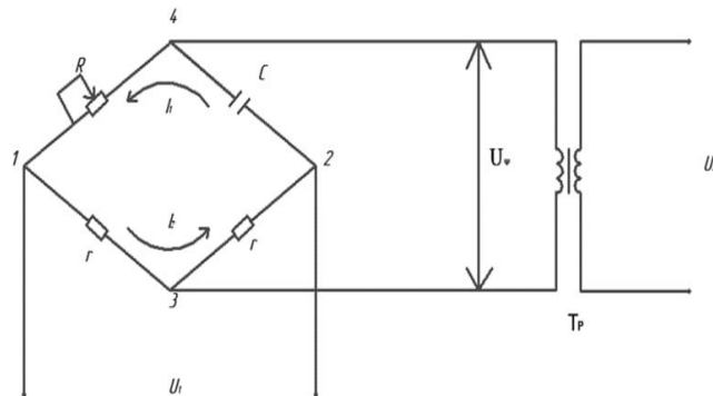
Рис.2 Схема питания одной из групп электродов с фазорегулятором.
