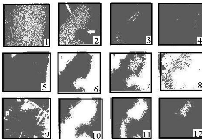
Рис. 1. Характерные магнитооптические картины неоднородных магнитных состояний индикаторной пленки, совмещенной с пленкой ВТСП, во внешнем магнитном поле, перпендикулярном ее поверхности ( T = 35 K).
