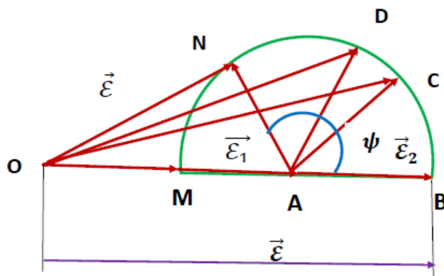
Рис.4. Круговая диаграмма напряженностей электрического поля в точках пересечения электродов.
