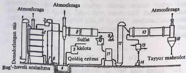
7.6-rasm. Donadorlangan misdan mis kuporosi ishlab chiqarish sxemasi: 1 va 12 – kovshli elevatorlar; 2 – yuvuvchi minora; 3 – bir xil darajali bak; 4 – qoldiq eritma yig'gichi; 5 – sulfat kislota uchun sarflash baki; 6 va 7 – markazdan qochma nasoslar; 8 – aylanuvchi kristallizator; 9 va 14 – ventilatorlar; 10 – aralashtirgichli yig'gich; 11 – sentrifuga; 13 – quritgich; 15 – havo isitgichi; 16 – tayyor mahsulot bunkeri.
