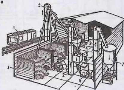
6.24-rasm. Tukoaralashtirish qurilmasining umumiy ko'rinishi (AQSH): 1 — temir yo'l vagoni; 2 — elevatorlar; 3 — omborlar bo'limasi; 4 — alohida o'g'itlar taqsimlagich bunkerlari; 5 — aralashtiriladigan o'g'itlar me'yorlashtirgich bunkerlari; 6 — barabanli aralashtirgich; 7 — tayyor aralashma uchun bunker.
