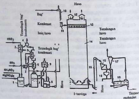
2.8-rasm. «Ikl» firmasi usuli bo'yicha donadorlangan ammiakli selitra ishlab chiqarish sxemasi: 1 – qattiq komponentlarni eritish idishi; 2 – filtr; 3,5 – isitgichlar; 4 – kondensator; 6 – suyuq ammiak bug'latgich; 7 – neytrallagich; 8 – qo'shimcha neytrallagich; 9 – bak; 10 – bug'latish jihozi; 11 – yig'gich bak; 12 – ventilatorlar; 13 – suyuqlarni tomchilatgich; 14 – donadorlash minorasi; 15 – elevator; 16 – elak; 17 – siklon; 18 – tegirmon; 19 – sovitgich jihozi.
