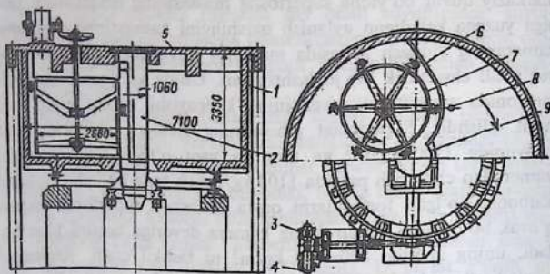
3.21-rasm. Uzluksiz ishlaydigan superfosfat kamerasi: 1 – kameraning silindrik korpusi; 2 – markaziy quvur; 3 – elektromotor; 4 – reduktor; 5 – kamera qopqog‘i; 6 – to‘siq; 7 – frezer; 8 – suspenziya tushish joyi; 9 – eksentrik.
