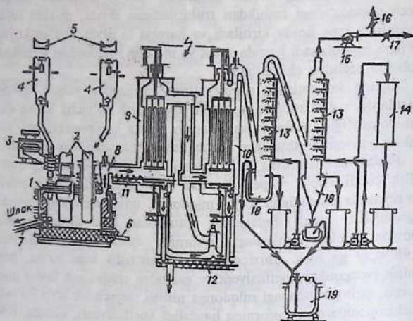
3.12-rasm. SARIQ fosfor ishlab chiqarish tasviri: 1 – elektropech; 2 – elektrodlar; 3 – transformator; 4 – yuklash bunkeri; 5 – transportyor; 6 – ferfosfor cho'michli quygichi; 7 – shlak juri; 8 – gazyig'ich; 9, 10 – elektrofiltrlar; 11, 12 – chang uchun shneklar; 13 – kondensatorlar; 14 – bug'ejeksiyal qurilma; 15 – gaz haydagich; 16 – gazni yoqish quvuri; 17 – gaz o'tkazish quvuri; 18 – suyuq fosforni yig'gich; 19 – suyuq fosforni saqlagich.
