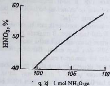
2.2-rasm. Nitrat kislotasini gaz holidagi ammiak bilan neytrallash issiqligi — q (atmosfera bosimi va 180°Cda).
