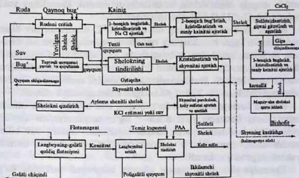
4.7-rasm. Prikarpat polimineral rudasini qayta ishlash sxemasi.
