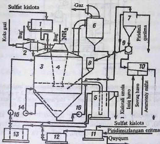
2.23-rasm. Ammoniy sulfat ishlab chiqarishning saturatorli usuli tasviri: 1 – sulfat kislotasi uchun bak; 2 – koks gazi uchun qizdircich; 3 – saturator; 4 – barbotyor; 5 – aylanuvchi eritma uchun bak; 6 – kislotatutgich; 7 – kristall yig'gich; 8 – eritma yig'gich; 9 – sentrafuga; 10 – «qaynovchi qatlam»li quritgich; 11 – piridinsizlantirilgan eritma uchun rezervuar; 12 – kislotali eritma uchun yig'gich; 13 – eritma uchun rezervuar; 14,15 – markazdan qochma nasoslar.
