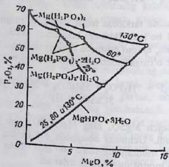
3.18-rasm. 25, 80 va 130^\circ\text{C} haroratdagi \text{MgO}-\text{P}_2\text{O}_5-\text{H}_2\text{O} sistemasida eruvchanlik izotermsi: ikkita qattiq fazali muvozanatdagi eritmaning tarkibi nuqtalar bilan belgilangan.
