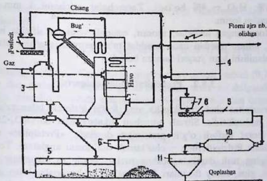
3.39-rasm. Siklonli kamerada ftorsizlangan fosfatlar ishlab chiqarish sxemasi:
