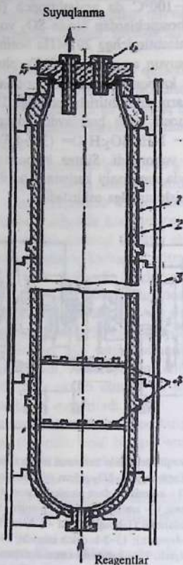
2.20-rasm. Karbamid sintez kolonnasi. 1 - korpus; 2 - himoya qatlami; 3 - himoya qatlami nazorat kollektori; 4 - panjara; 5 - qopqoq; 6 - termopara uchun shtutser.
