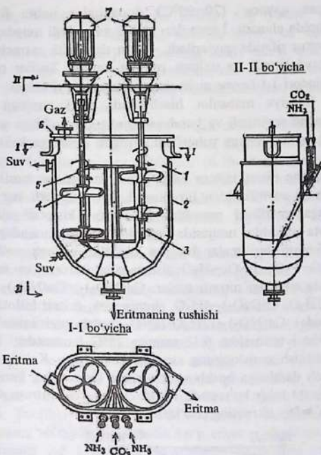
6.17-rasm. Reaktor-ammoniylashtirgish: 1 — korpus; 2 — sovitish g'ilofi; 3 — val; 4 — aralashtirgich kurakchasi; 5 — to'siq; 6 — qopqog'; 7 — elektrodvigatel; 8 — reduktorlar.
