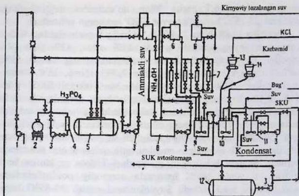
6.21-rasm. Suyuq kompleks o'g'itlar ishlab chiqarish sxemasi: 1 – vakuum-nasos; 2 – temir yo'l sisternasi; 3 – markazdan qochma nasoslar; 4 – sifonli qurilma; 5 – fosfat kislota saqlagichi; 6 – quyuvchi bak; 7 – rotametrlar; 8 – ammiakli suv bilan ta'minlash baki; 9 – fosfat kislota neytrallagichi; 10 – tuzlarni eritish uchun jihoz; 11 – oxirgi aralashtirish (aralashtirishni tugallash) uchun jihoz; 12 – SKH ombori; 13, 14 – ta'minlagichli bunker.
