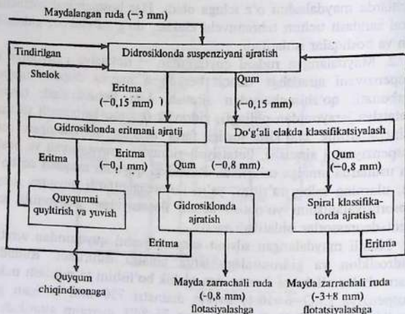
4.2-rasm. Silvinit rudasini quyqumsizlantirish sxemasi.
