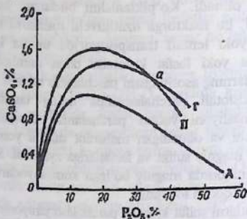
3.14-rasm. 80^{\circ}\text{C} da fosfat kislotada kalsiy sulfatning eruvchanlik izotermasi: A – angidrit; P – yarimgidrat; G – gips.
