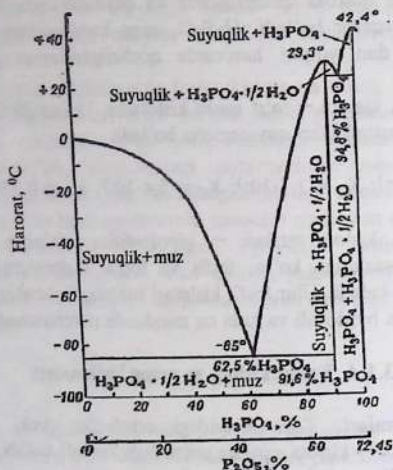
3.1-rasm. \text{H}_3\text{PO}_4 - \text{H}_2\text{O} sistemasining holat diagrammasi.
