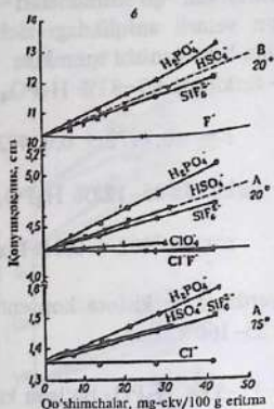
3.3-rasm. Kationlar (a) va anionlar (b) ishtirokida fosfat kislotali eritmalar qovushqoqligining o'zgarishi. Boshlang'ich kislotada: A – 30% P_2O_5 va 2% H_2SO_4 ; V – 43% P_2O_5 va 3% H_2SO_4 ; S – 54% P_2O_5 va 4% H_2SO_4 bo'ladi.
