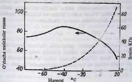
7.1-rasm. Vodorod ftorid bug'ining o'rtacha molekular massasi va to'yingan bug' bosimi
