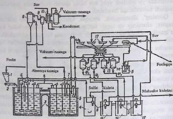
3.25-rasm. Digidratli usulda ekstraksiya fosfat kislota ishlab chiqarish sxemasi: 1 - fosfatli xomashyo uchun bunker; 2 - og'irlik o'lchov me'yorigishi; 3 - ikki bankali ekstraktor; 4 - sulfat kislota saqlagich; 5 - botirma nasoslar; 6 - sulfat kislota saqlagich; 7 - sirkulatsiyali botirma nasos; 8 - bug'latgich; 9 - tomchi ushlagich; 10 - kondensator; 11 - barbotajli neytrallagich; 12 - karusel vakuu-filtrning tarmovlari; 13 - separatorlar; 14 - filtrli to'qima regeneratsiyasidan hosil bo'luvchi suspenziyaning oraliq yig'gichi; 15, 16, 17 - birinchi (asosiy) filtrat uchun (15), aylanma fosfat kislota uchun (16), yuvindi filtrat uchun (17) barometrik yig'gichlar.
