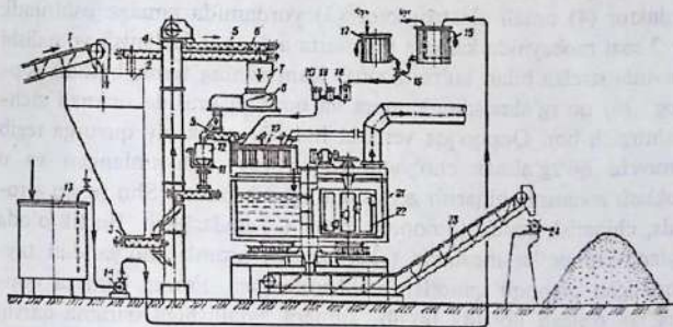
3.19-rasm. Superfosfat ishlab chiqarish sxemasi: 1 – apatit konsentrati uchun transportyor; 2 – bunker; 3 – shnekli ta'minlagich; 4 – cho'michli elevator; 5, 9 – shneklar; 6 – ortiqcha apatit konsentrati uchun qaytuvchi shnek; 7 – me'yorlashtirgich bunker; 8 – me'yorlashtirgich; 10 – aralashtirgich; 11 – o'lovli me'yorlashtirgichni tekshirish uchun nazorat tarozisi; 12 – nazorat tarozisi uchun bunker; 13 – sulfat kislota uchun rezervuar; 14 – markazdan qochma kislotali nasos; 15 – kislota uchun bak; 16 – kislota aralashtirgich; 17 – suv uchun bak; 18 – minerali sulfat kislotali suyultirishda ajraladigan azot oksidlari uchun gaz ajratgich; 19 – kislota uchun konsentratomer; 20 – tirqishli kislota sarflagich; 21 – superfosfat kamerasi; 22 – frezer; 23 – kamerali superfosfat transportyori; 24 – supyerfosfatni ombonga tashlagich.
