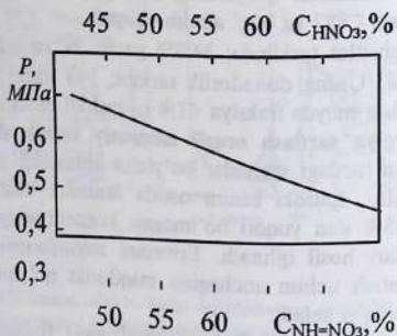
2.9-rasm. Neytrallagichdagi bosim, ammiakli selitra konsentratsiyasi va boshlang'ich nitrat kislota orasidagi o'zaro bog'liqlik (ishchi harorat 180°C).
