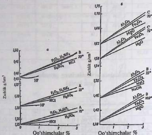
3.2-pasm. Kislotalar (a), oksidlar va ishqorlar (b) ishtirokida fosfat kislotali eritmalr zichligining o'zgarishi. Boshlang'ich kislotalar: A—30% P_2O_5 va 2% H_2SO_4 ; B—43% P_2O_5 va 3% H_2SO_4 ; C—54% P_2O_5 va 6% H_2SO_4 bo'ladi.
