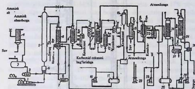
2.19-rasm. Suyuqlik retsiklida karbamid ishlab chiqarish sxemasi (sintez va suyuqlanish distillatsiyasi). 1 — \text{SO}_2 uchun to'rt bosqichli kompressor; 2 — suyuq ammiak tankeri; 3 — ammiak uchun plunjerli nasos; 4 — 1-bosqich kondensatori; 5 — sintez kolonnasi; 6 — aralashtirgich; 7 — plunjerli nasos; 8 — yuvuvchi kolonna; 9 — rektifikatsiya kolonnasi (1-bosqichi); 11 — 1-bosqich separatori; 12 — rektifikatsiya kolonnasi (2-bosqich); 13 — 2-bosqich isitgichi; 14 — 2-bosqich separatori; 15 — vakuum-bug'latgich; 16 — karbamid eritmasi uchun yig'gich; 17 — moy ajratgich; 18 — markazdan qochma nasos; 19 — kondensator; 20 — vakuum-nasos; 21 — 2-bosqich kondensatori; 22 — rezervuar; 23 — markazdan qochma nasos; 24 — absorber; 25 — ammoniy karbonat tuzlari eritmasi uchun yig'gich; 26 — desorber; 27 — sovitgich; 28 — issiqlik almashtirgich; 29 — markazdan qochma nasoslar.
