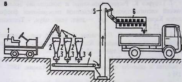
6.26-rasm. Kuban qishloq xo'jaligi instituti qurilmasi (Rossiya). 1 – yuklovchi mashina; 2 – komponentlar uchun bunkerlar; 3 – me'yorlashtirgichlar; 4 – transportyor; 5 – elevator; 6 – aralashtirgich.
