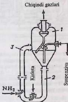
6.10-rasm. Tezkor ammoniylashtiruvchi bug'latgich (TAB). beriladi, 1- va 2-qobiqlarda esa jarayonda hosil bo'ladigan bug' ishlatiladi.
