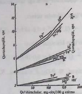
3.3-rasm. Kationlar (a) va anionlar (b) ishtirokida fosfat kislotali eritmalar qovushqoqligining o'zgarishi. Boshlang'ich kislotada: A – 30% P_2O_5 va 2% H_2SO_4 ; V – 43% P_2O_5 va 3% H_2SO_4 ; S – 54% P_2O_5 va 4% H_2SO_4 bo'ladi.
