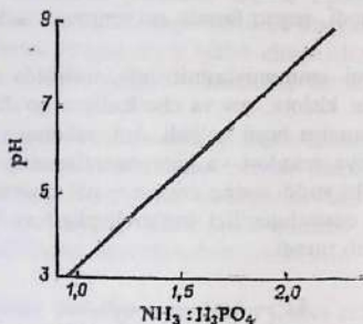
6.6-rasm. 65\text{--}75^\circ\text{C} haroratdagi ammoniy fosfatlar to'yingan eritmaları pH qiymatining \text{NH}_3:\text{H}_3\text{PO}_4 molar nisbatiga bog'liqligi.
