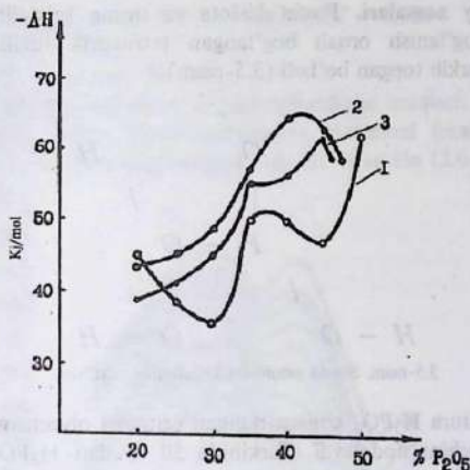
3.4-rasm. Fosfat kislotali eritma bug'lanish issiqqligining eritma konsentratsiyasiga bog'liqligi: 1 - H_3PO_4, H_2O ; 2 - H_3PO_4, MgSO_4 \cdot 7H_2O, H_2O ; 3 - H_3PO_4, MgSO_4 \cdot 7H_2O, NH_4NO_3, H_2O
