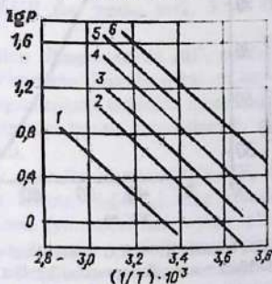
7.2-rasm. Ftorid kislota suvli eritmasi ustidagi HF ning bug' bosimi (P, kPa):HF miqdori, %: 1 - 41,2; 2 - 50,9; 3 - 55,1; 4 - 60,52; 5 - 65,45; 6 - 70,23.
