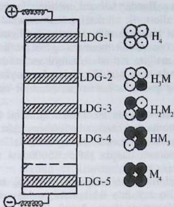
9-rasm. Laktatdegidrogenazaning poliakrilamid gelida elektroforez qilinganda izofermentlarga ajralishi. LDG-1, 2, 3, 4, 5—laktatgidrogenaza izofermentlarining elektroforegrammasi.
