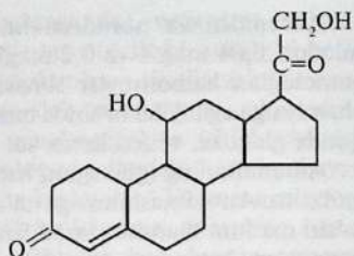
Kortikosteron
