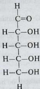
Riboza
