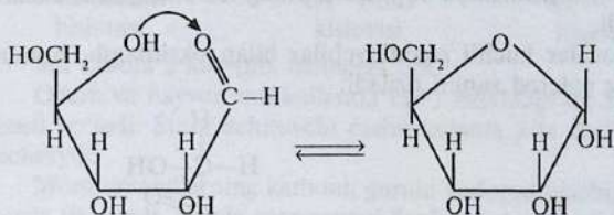
A. Ribozaning (aldegid) davriy shakli
