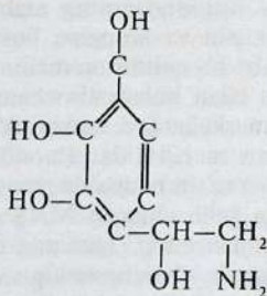
Noradrenalin
