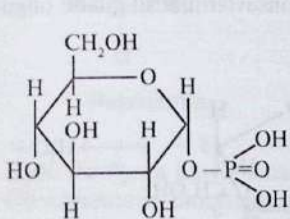
Glukoza-1-fosfat
