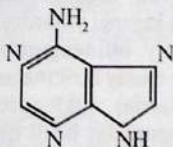
adenin
