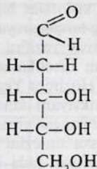
Dezoksiriboza
