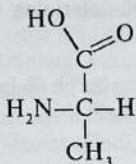
L-alanin
