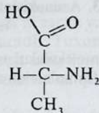
D-alanin
