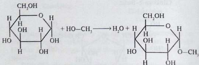
Glukoza
