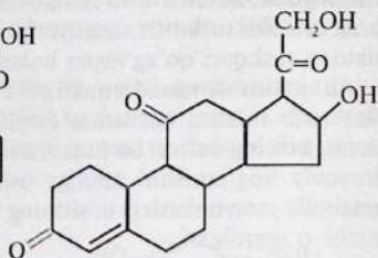
Kortizon
