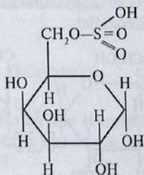
Galaktoza-6-sulfat
