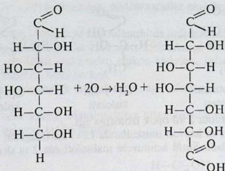
Galaktoza
