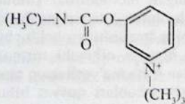
Neostegmin
