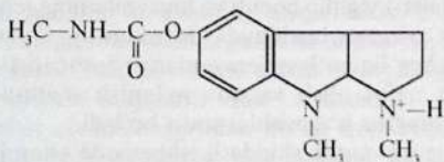
Ezerin
