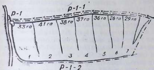
5-чи расм. Колхозда Р—1—1 ариғидан сув бериладиган участкаларнинг бир қисми.
